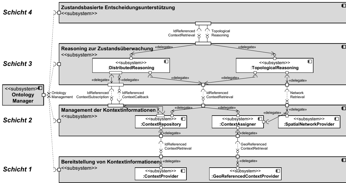
Abbildung 7.1.: Funktionale Schichten der integrierenden Systemarchitektur.
