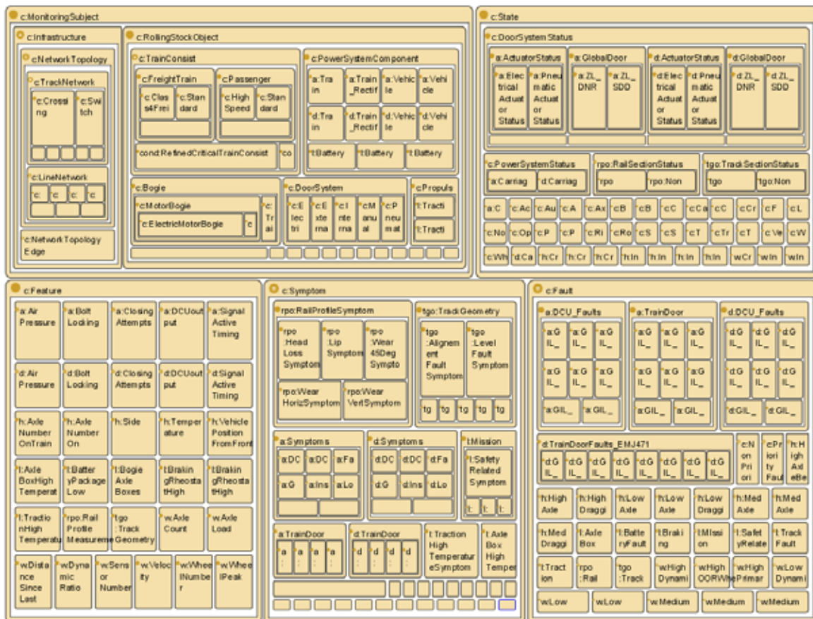
Abbildung 7.5.: Überblick über ausgewählte Überwachungsobjekt-, Zustands-, Merkmals-, Symptom- und Fehlerkonzepte der Ontologie für Zustandsüberwachung bei Schienennetzen. Die Darstellung wurde mit dem Ontologie-Editor Protégé generiert: Rechtecke repräsentieren Konzepte, ihre Schachtelung stellt die Konzeptinklusion dar.
