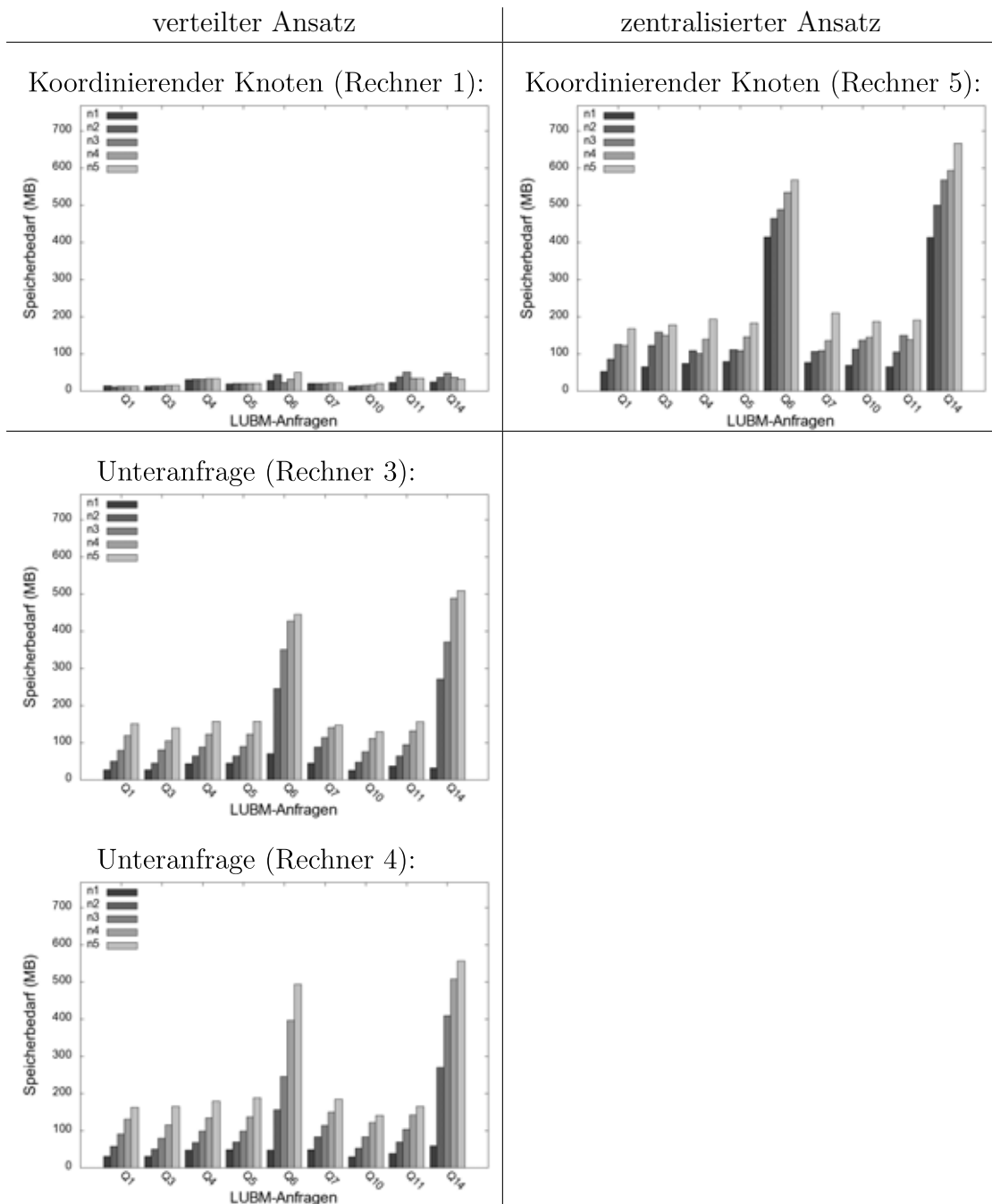
Abbildung 5.13.: Gegenüberstellung des Speicherbedarfs für die LUBM-Anfragen im verteilten (links) und zentralisierten Fall (rechts) mit steigender Größe der Wissensbasen. Für den verteilten Fall ist außerdem jeweils der Speicherbedarf der beteiligten Knoten auf den Rechnern 3 und 4 dargestellt.
