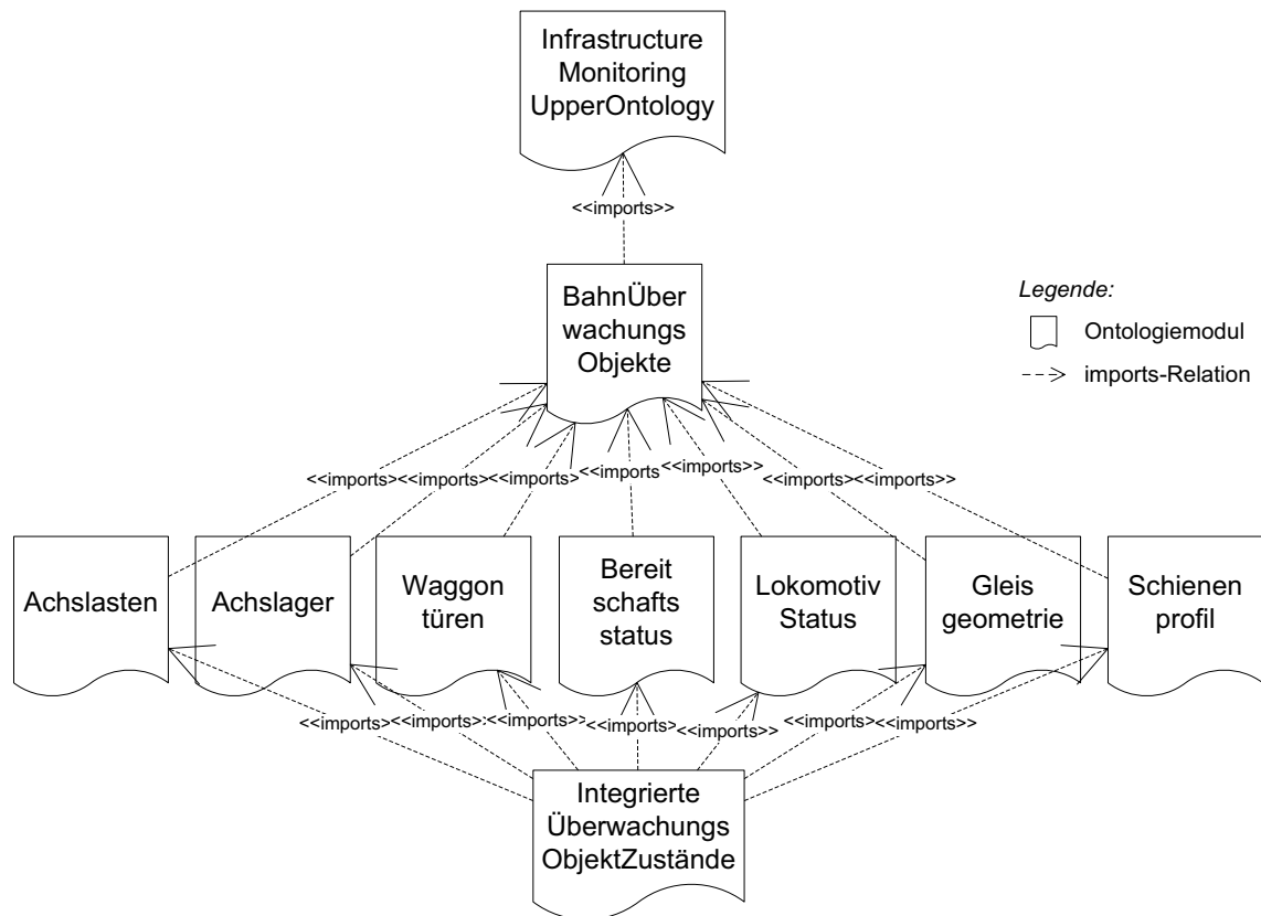
Abbildung 7.4.: Überblick über die Architektur der Ontologie für Zustandsüberwachung bei Schienennetzen.
