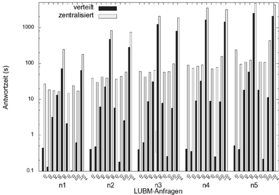
Abbildung 5.11.: Direkte Gegenüberstellung der Antwortzeiten für die LUBM-Anfragen mit steigender Größe der Wissensbasen.
