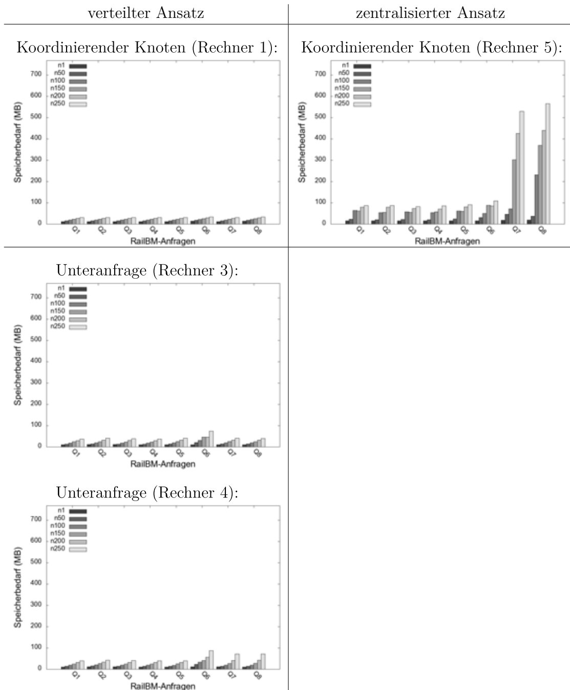
Abbildung 5.21.: Gegenüberstellung des Speicherbedarfs für die RAILBM-Anfragen im verteilten (links) und zentralisierten Fall (rechts) mit steigender Größe der Wissensbasen. Für den verteilten Fall ist außerdem jeweils der Speicherbedarf der beteiligten Knoten auf den Rechnern 3 und 4 dargestellt.
