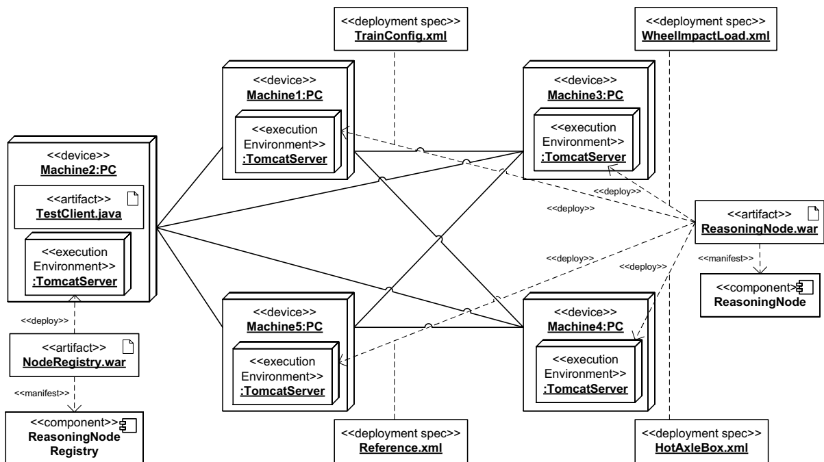
Abbildung 5.9.: Testaufbau für die experimentelle Evaluierung.
