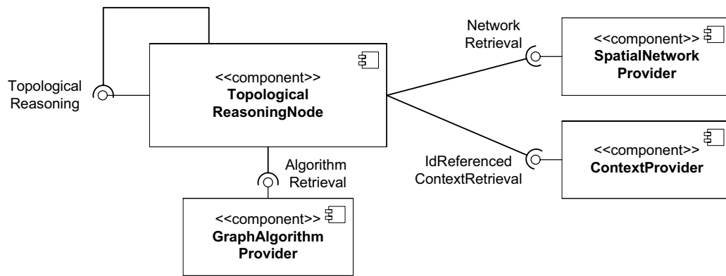
Abbildung 6.12.: Komponentenarchitektur für Reasoning mit Topologiebezug.
