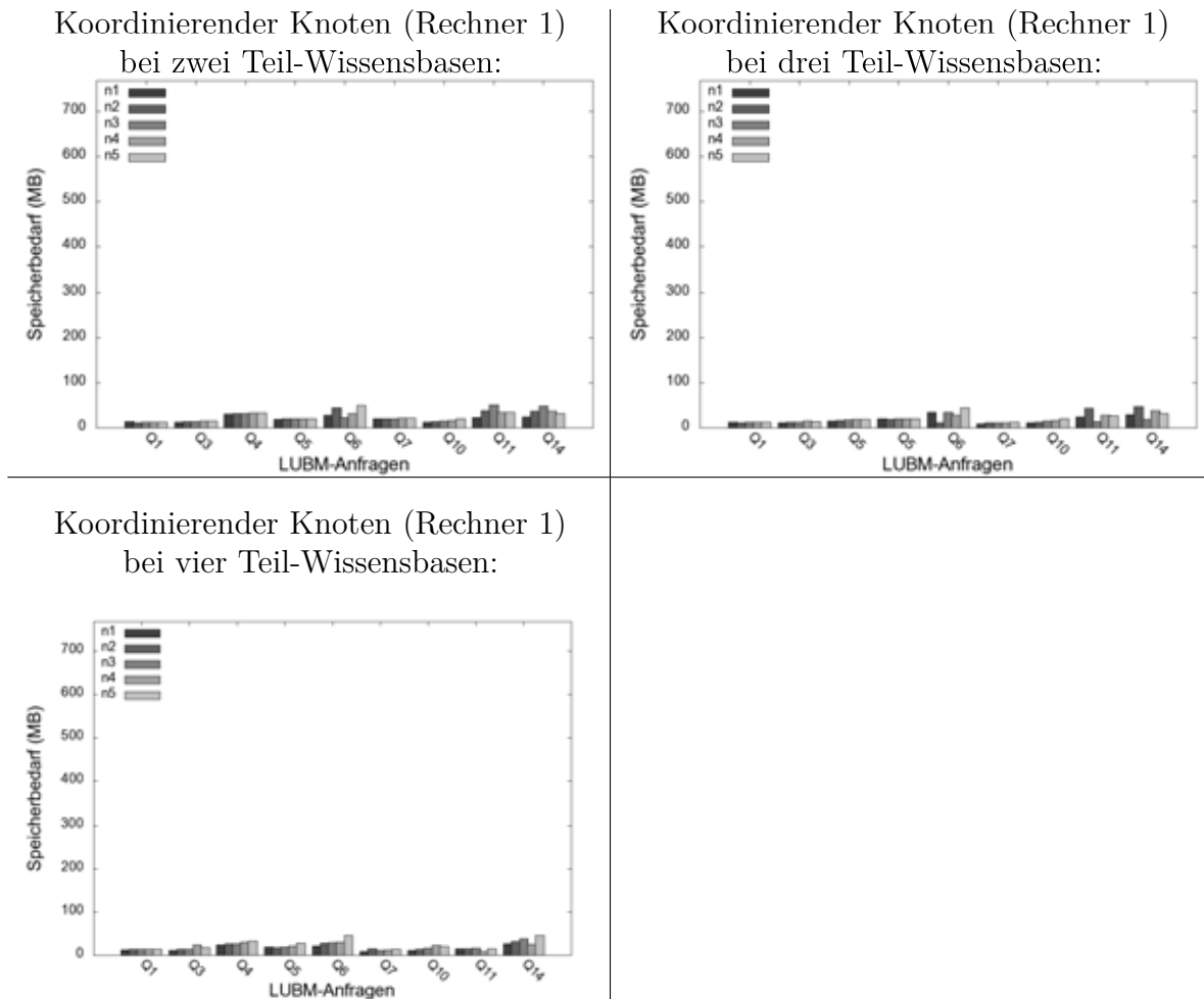
Abbildung 5.15.: Gegenüberstellung des Speicherbedarfs im verteilten Fall beim koordinierenden Knoten für die LUBM-Anfragen bei zwei bis vier Teil-Wissensbasen.
