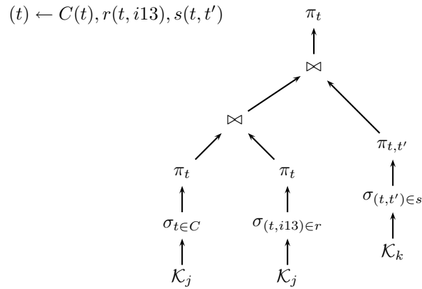
Abbildung 5.4.: Beispiel für einen relationalen Operatorbaum.
