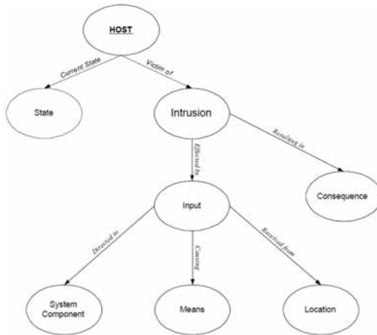
Abbildung 4.1.: Ontologie zur Eindringlingserkennung in Rechnernetzen [UJFP04].
