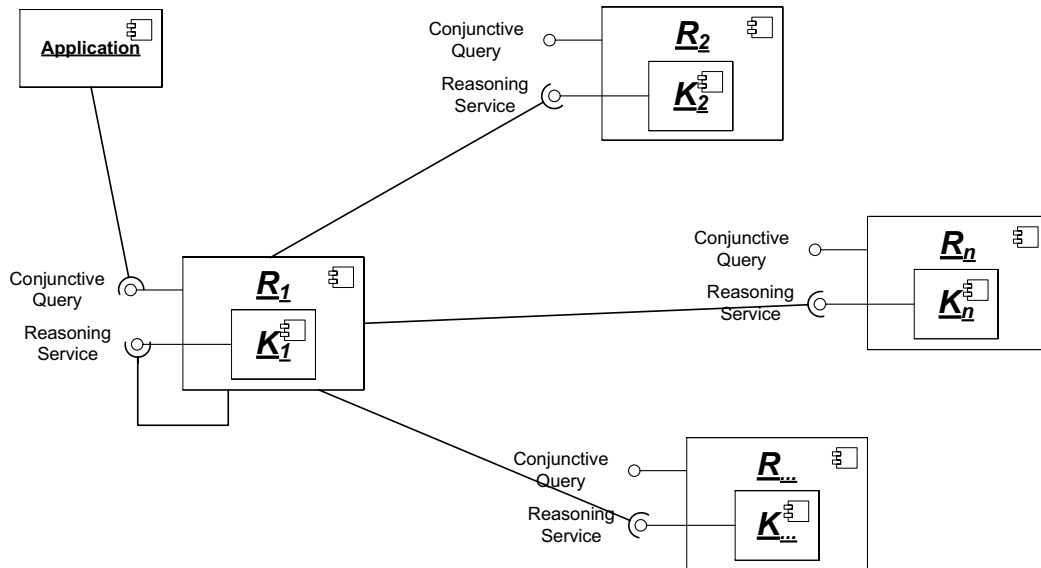
Abbildung 5.1.: Verteiltes Reasoning-System \mathfrak{R} mit Reasoning-Knoten R_j und Teil-Wissensbasen \mathcal{K}_j .
