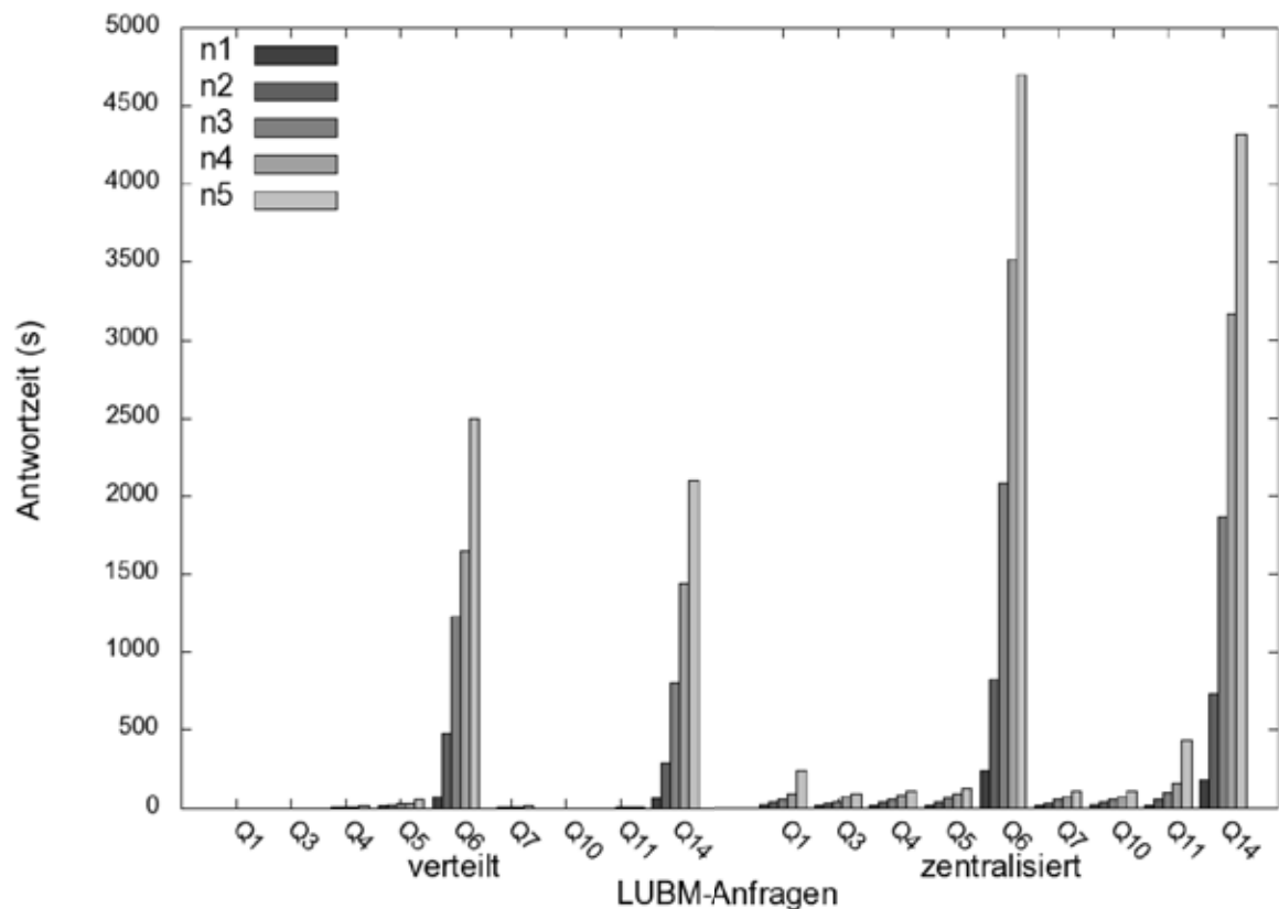
Abbildung 5.10.: Gegenüberstellung der Antwortzeiten für die LUBM-Anfragen mit steigender Größe der Wissensbasen im verteilten (links) und zentralisierten Fall (rechts).
