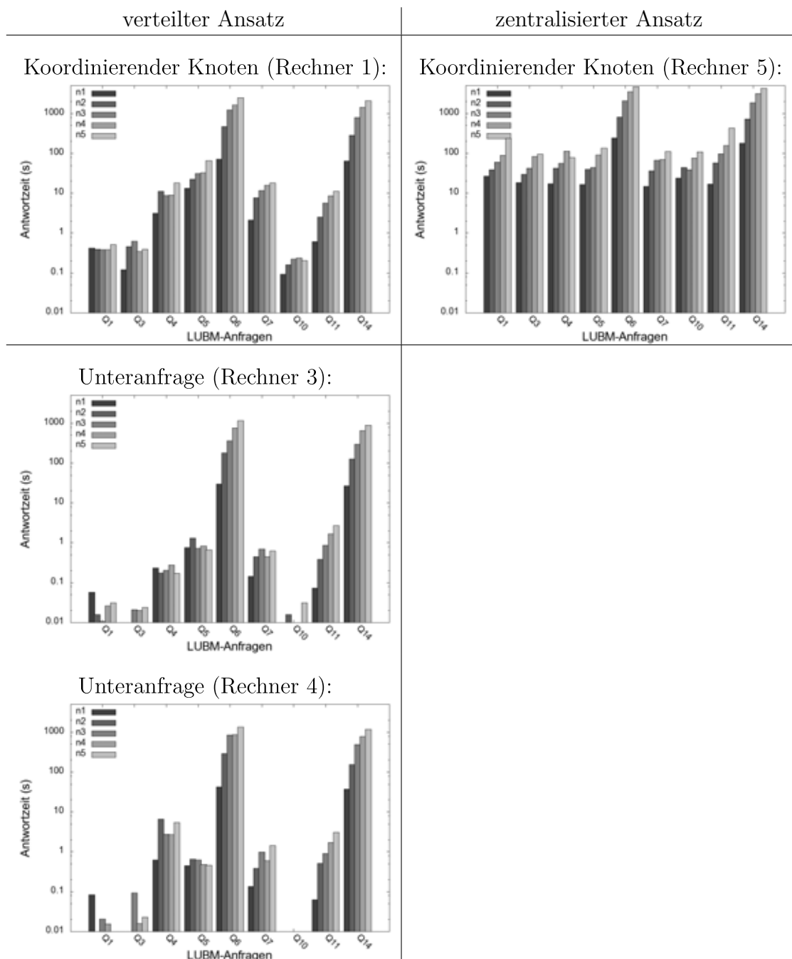
Abbildung 5.12.: Gegenüberstellung der Antwortzeiten für die LUBM-Anfragen im verteilten (links) und zentralisierten Fall (rechts) mit steigender Größe der Wissensbasen. Für den verteilten Fall sind außerdem die Antwortzeiten für die beteiligten Knoten auf den Rechnern 3 und 4 dargestellt.
