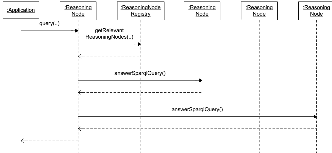
Abbildung 5.6.: Beispiel für Interaktionen zwischen den Komponenten des Frameworks.
