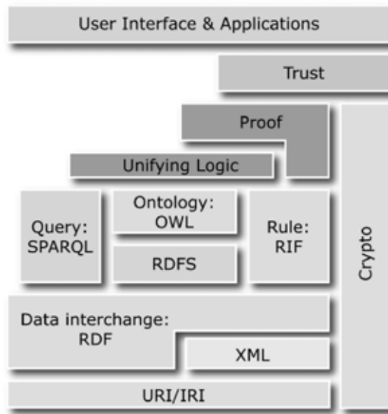
Abbildung 3.8.: „Schichttorte“ des Semantic Web [SW08].
