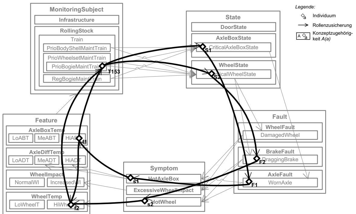
Abbildung 4.7.: Implizite Aussagen in der Wissensbasis, die gefolgert werden können.
