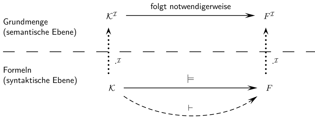
Abbildung 3.4.: Syntaktische und semantische Ebene bei logischen Formalismen.
