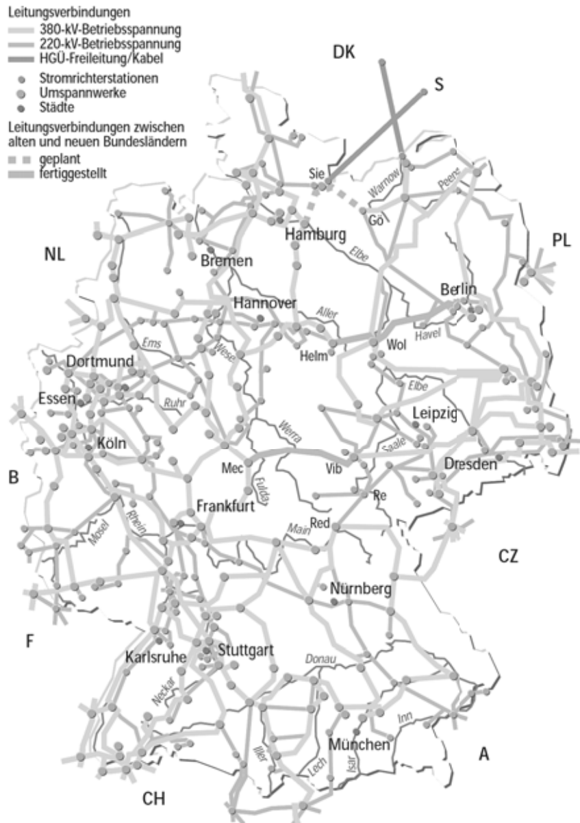
Abbildung 2.3.: Stromübertragungsnetz in Deutschland (Stand: 1. Januar 1996, nach [Sch05]).
