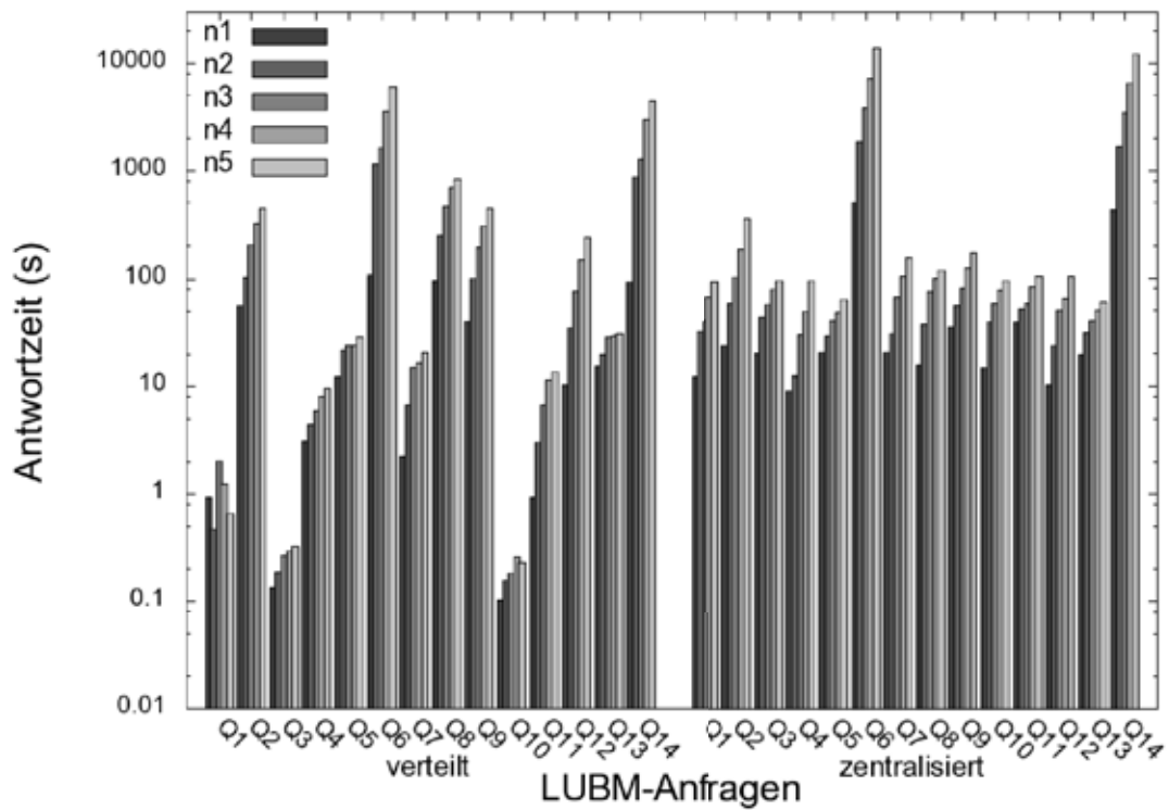
Abbildung A.2.: Gegenüberstellung der Antwortzeiten für alle LUBM-Test-Anfragen bei drei Teil-Wissensbasen.
