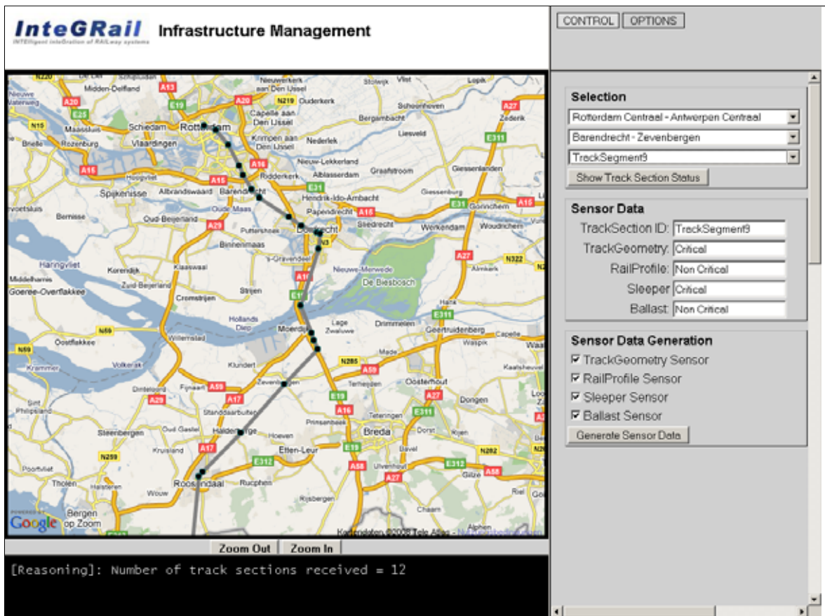
Abbildung 7.6.: Screenshot des Demonstrators für zustandsorientierte Instandhaltung des Schienennetzes [IGRP08]: In der links dargestellten Karte werden Gleisabschnitte ausgewählt. Rechts werden die verfügbaren Kontextinformationen und ein daraus abgeleiteter Gesamtzustand angezeigt. Zusätzlich kann der Ausfall bestimmter Kontextquellen simuliert werden, um zu demonstrieren, dass aufgrund der open world assumption dennoch keine falschen Ableitungen getroffen werden.
