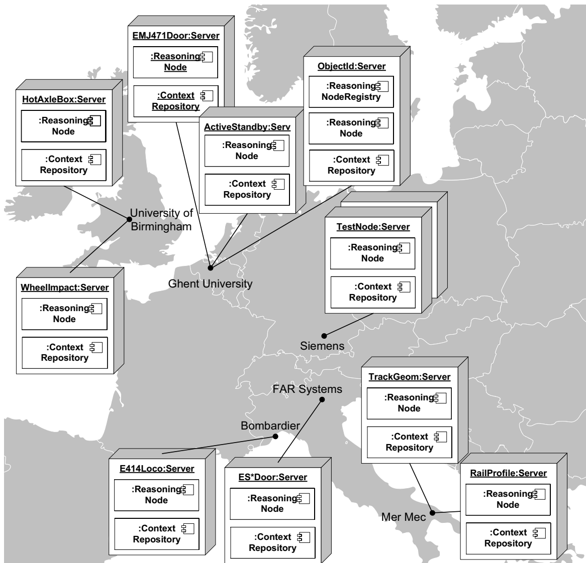
Abbildung 7.3.: Umsetzung von Schicht 2 und 3 der Systemarchitektur für Zustandsüberwachung im europäischen Schienennetz.
