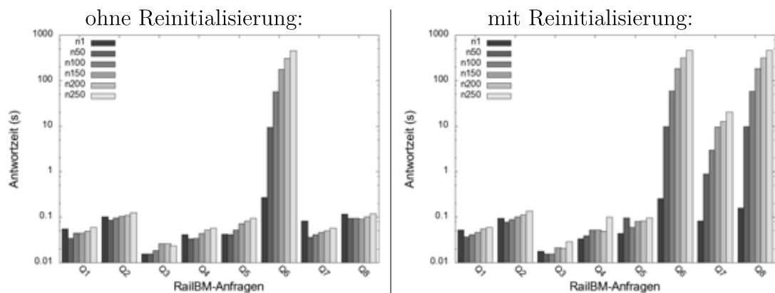
Abbildung 5.18.: Auswirkung der Reinitialisierung auf die Antwortzeiten für die RAILBM-Anfragen beim verteilten Ansatz.
