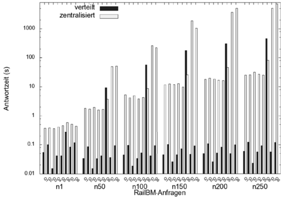
Abbildung 5.17.: Direkte Gegenüberstellung der Antwortzeiten für die RAILBM-Anfragen bei steigender Größe der Wissensbasen.
