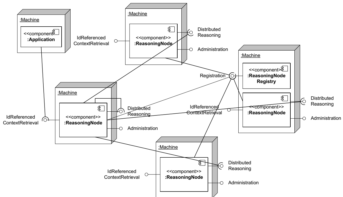
Abbildung 5.5.: Mögliche Verteilung der Komponenten zum Reasoning über verteilte Kontextinformationen.
