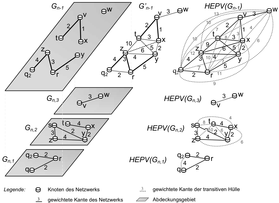
Abbildung 6.7.: Beispiele für die Erzeugung von hierarchisch kodierten Pfad-Sichten (nach [Mie07]).
