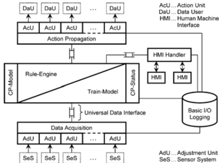
Abbildung 2.2.: Datenkonzentrator des Checkpoint-Systems [SM06].
