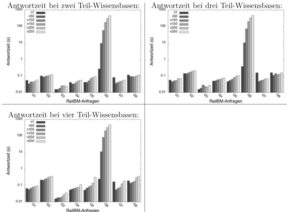
Abbildung 5.23.: Gegenüberstellung der Antwortzeiten im verteilten Fall für die RAILBM-Anfragen bei zwei bis vier Teil-Wissensbasen.
