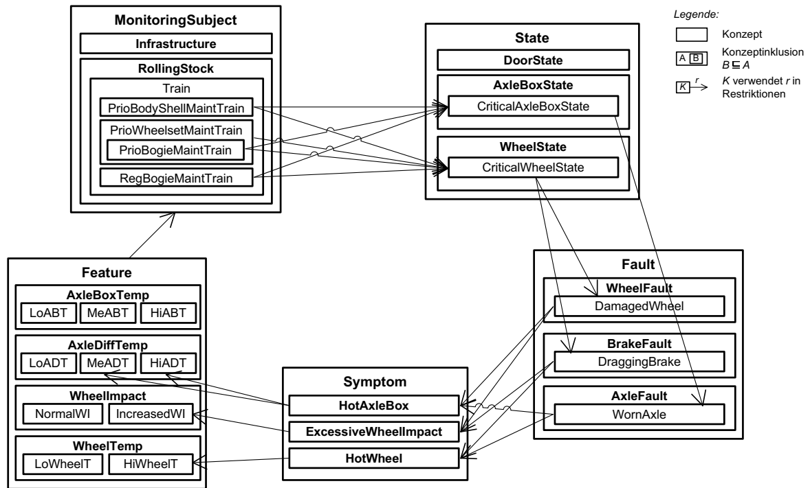
Abbildung 4.5.: Beispiele für den Einsatz des Entwurfsmusters zur Definition domänenspezifischer Merkmale, Symptome, Fehler, Zustände und Überwachungsobjekte.
