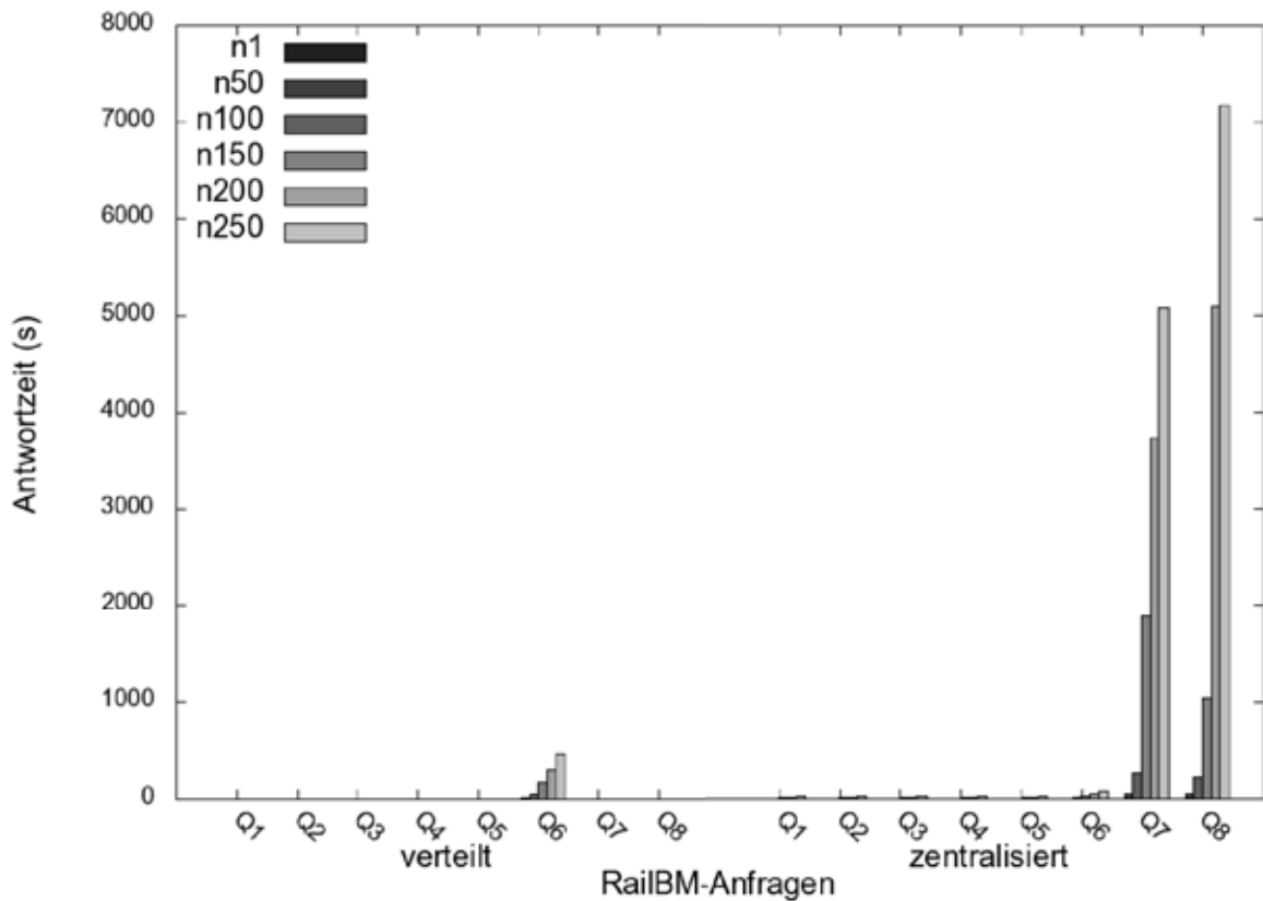
Abbildung 5.16.: Gegenüberstellung der Antwortzeiten für die RAILBM-Anfragen mit steigender Größe der Wissensbasen im verteilten (links) und zentralisierten Fall (rechts).
