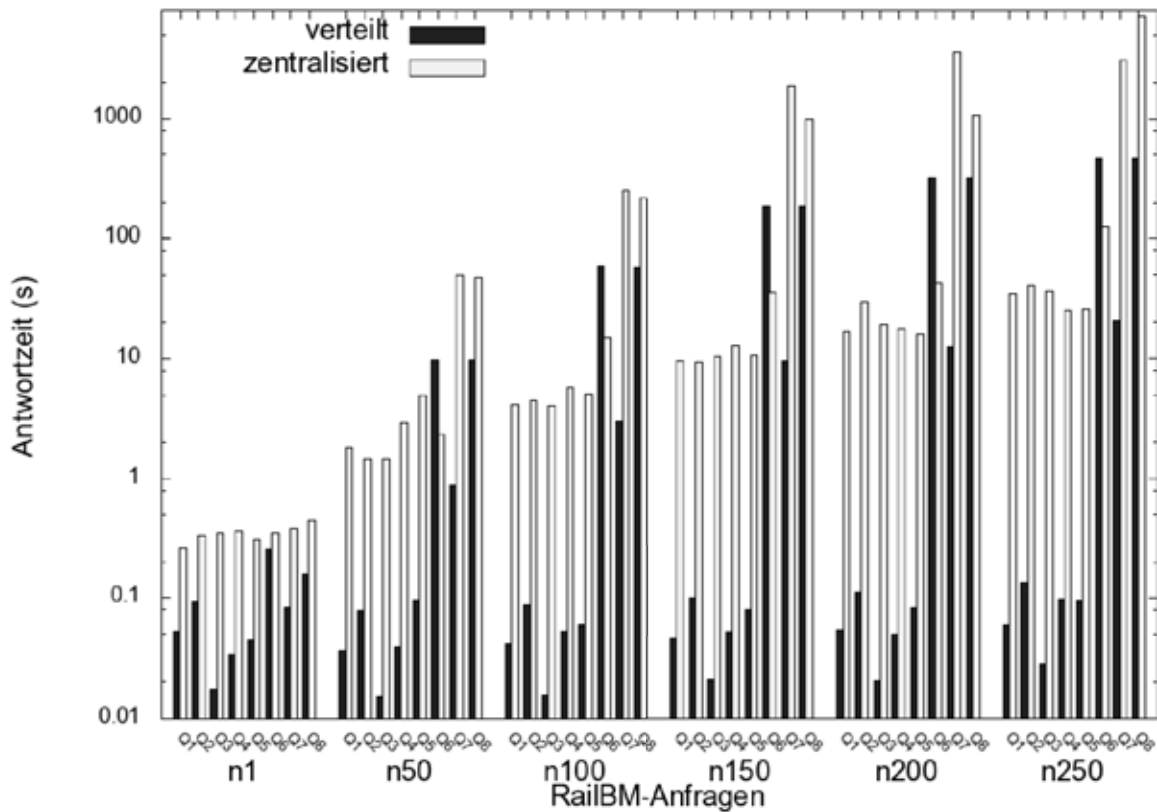
Abbildung 5.19.: Direkte Gegenüberstellung der Antwortzeiten für die RAILBM-Anfragen mit Reinitialisierung bei steigender Größe der Wissensbasen.
