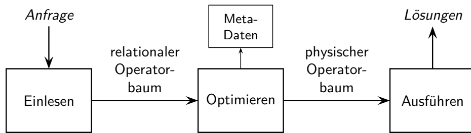
Abbildung 5.3.: Grundlegende Phasen der Anfragebearbeitung (nach [RG03]).
