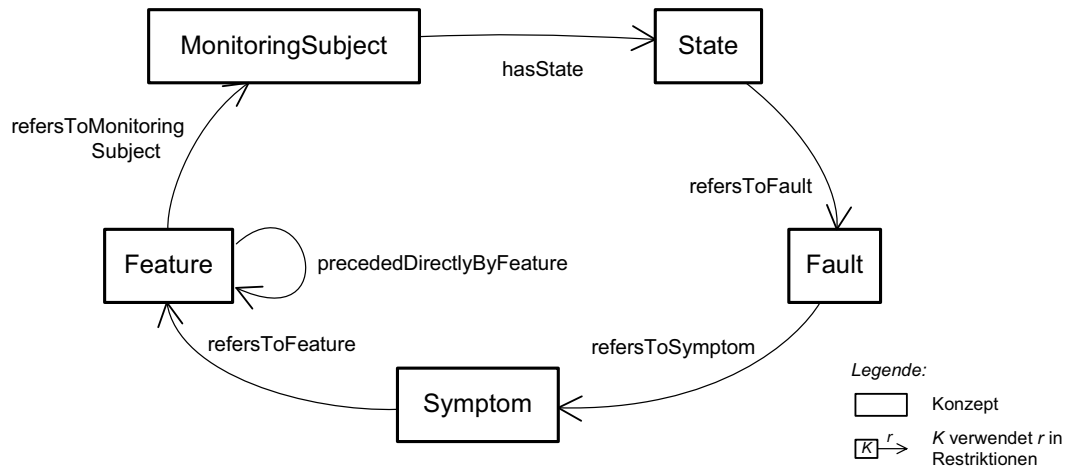
Abbildung 4.4.: Kernkonzepte und Zusammenhänge des Entwurfsmusters für Infrastrukturzustände.
