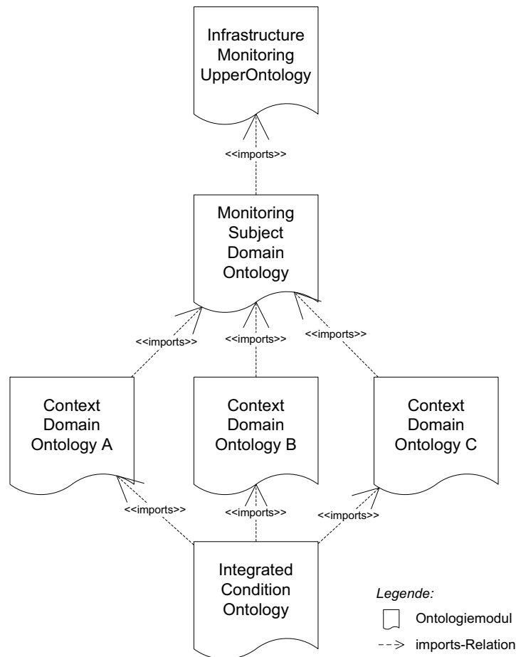
Abbildung 4.8.: Illustration des Architekturmusters zur Integration mehrerer Domänenontologien.
