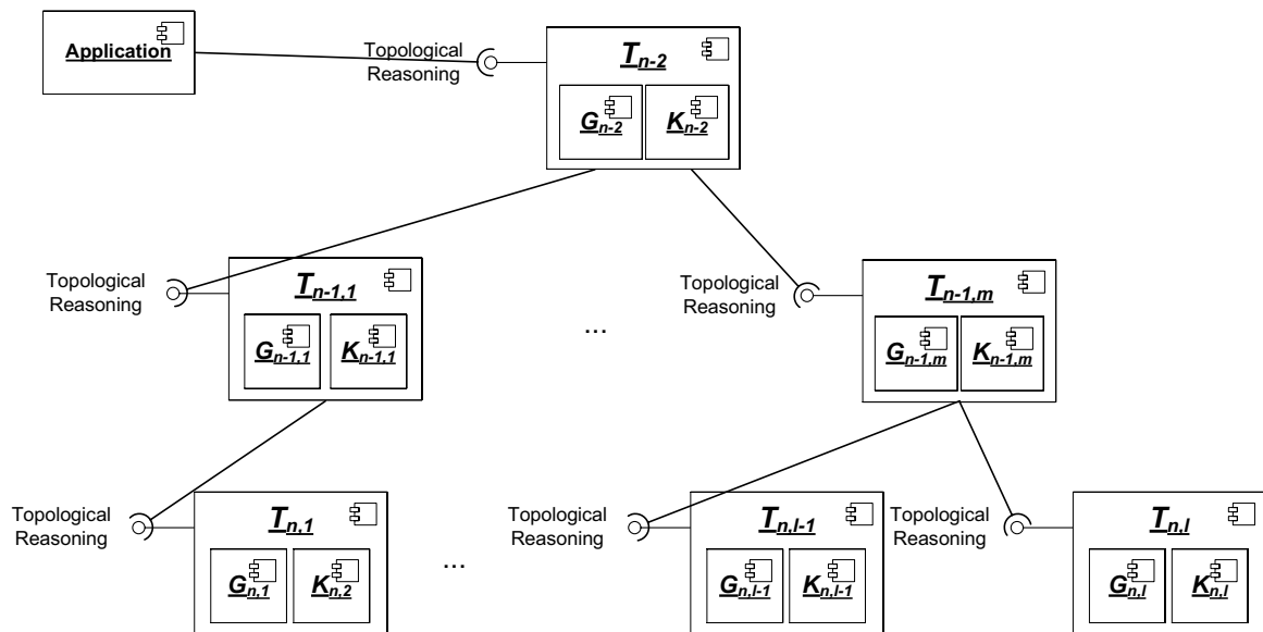
Abbildung 6.6.: Konzeptionelles topologiebezogenes Reasoning-System mit topologiebezogenen Reasoning-Knoten T_j , denen jeweils ein räumliches Teil-Netzwerk G_j und eine Wissensbasis K_j mit Kontextinformationen zu den Kanten und Knoten in G_j zugeordnet ist.
