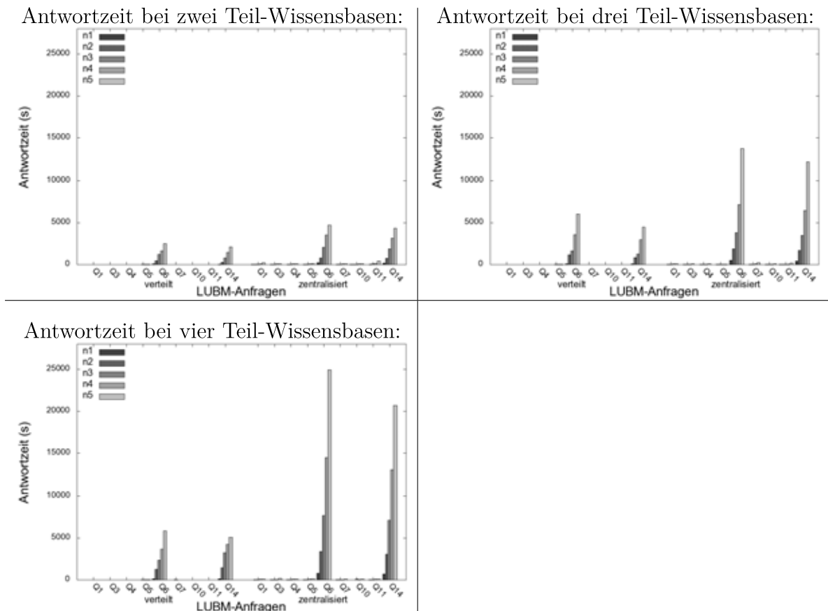
Abbildung 5.14.: Gegenüberstellung der Antwortzeiten im verteilten Fall für die LUBM-Anfragen bei zwei bis vier Teil-Wissensbasen.
