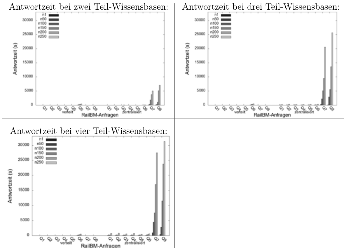
Abbildung 5.22.: Gegenüberstellung der Antwortzeiten im verteilten Fall für die RAILBM-Anfragen bei zwei bis vier Teil-Wissensbasen.
