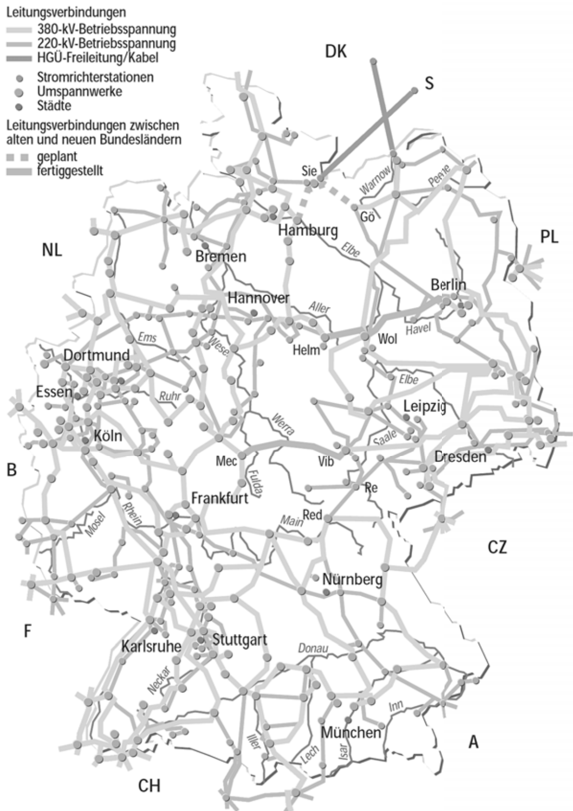
Abbildung 6.3.: Deutsches Stromverbundnetz (Stand: 1. Januar 1996, nach [Sch05]).
