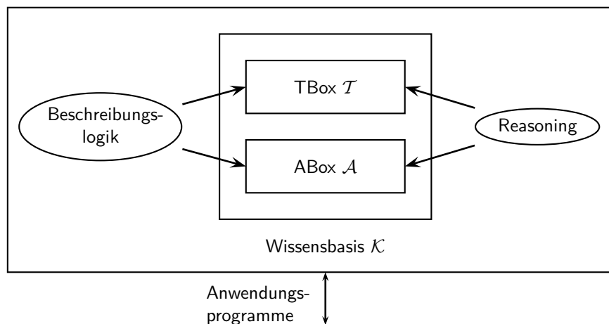
Abbildung 3.7.: Architektur eines beschreibungslogischen wissensbasierten Systems (nach [BCM + 03]).
