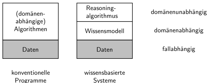
Abbildung 3.1.: Wissensbasierte Systeme und konventionelle Programme im Vergleich.
