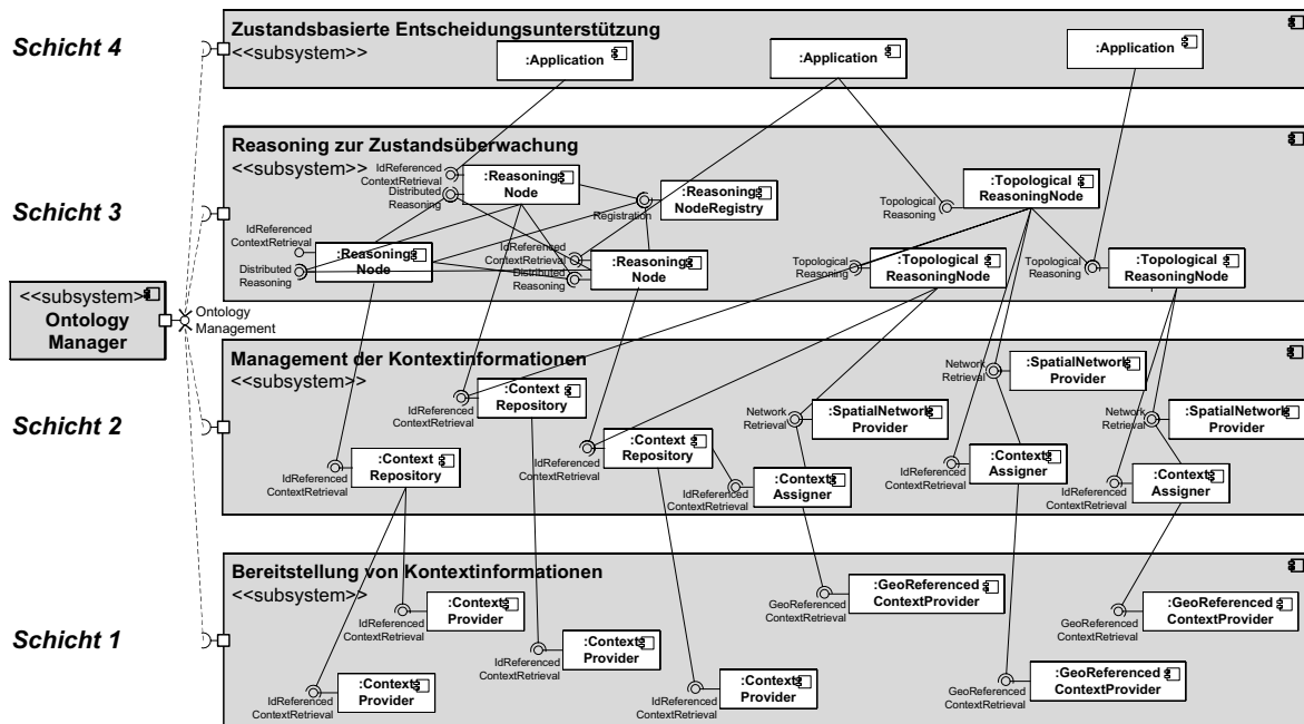
Abbildung 7.2.: Beispielhafte Realisierung der funktionalen Schichten mit den in dieser Arbeit eingeführten Komponenten.
