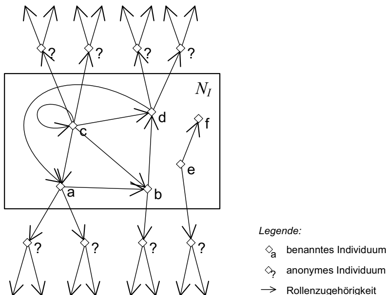
Abbildung 3.9.: Prinzipielle Struktur des Kompletierungswalds zu einer Wissensbasis.
