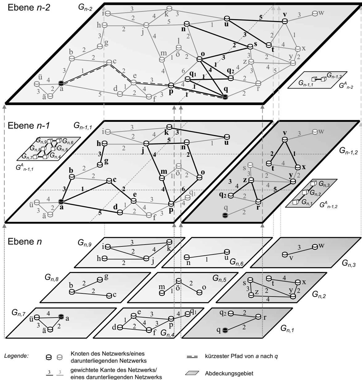
Abbildung 6.8.: Beispiel für eine Verfeinerungs-basierte Suche nach einem kürzesten Pfad von a in G_{n,7} nach q in G_{n,1} (nach [Mie07]).
