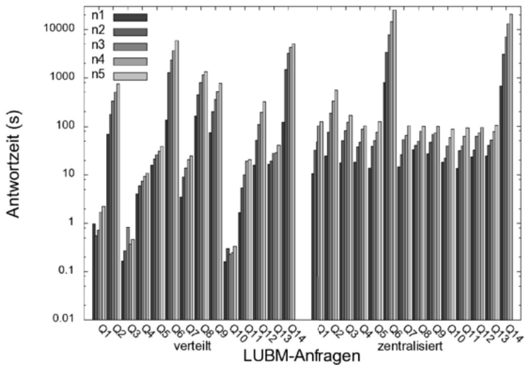
Abbildung A.3.: Gegenüberstellung der Antwortzeiten für alle LUBM-Test-Anfragen bei vier Teil-Wissensbasen.
