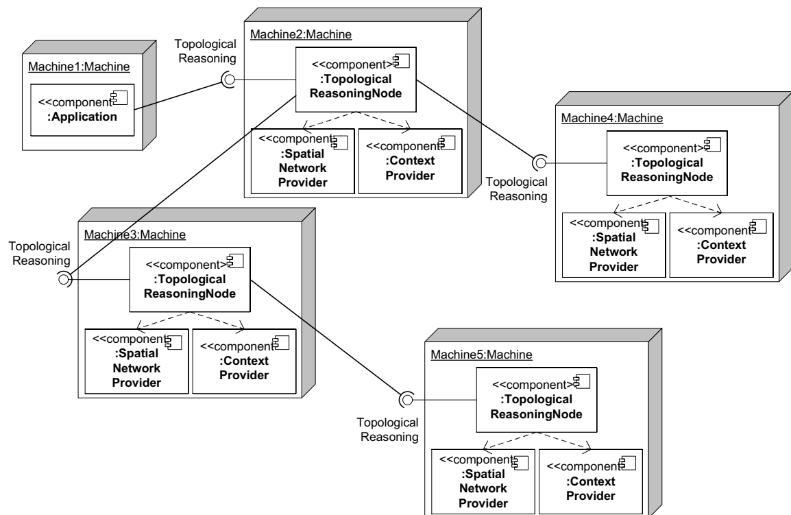
Abbildung 6.11.: Mögliche Verteilung der Komponenten zum Reasoning mit Topologiebezug.
