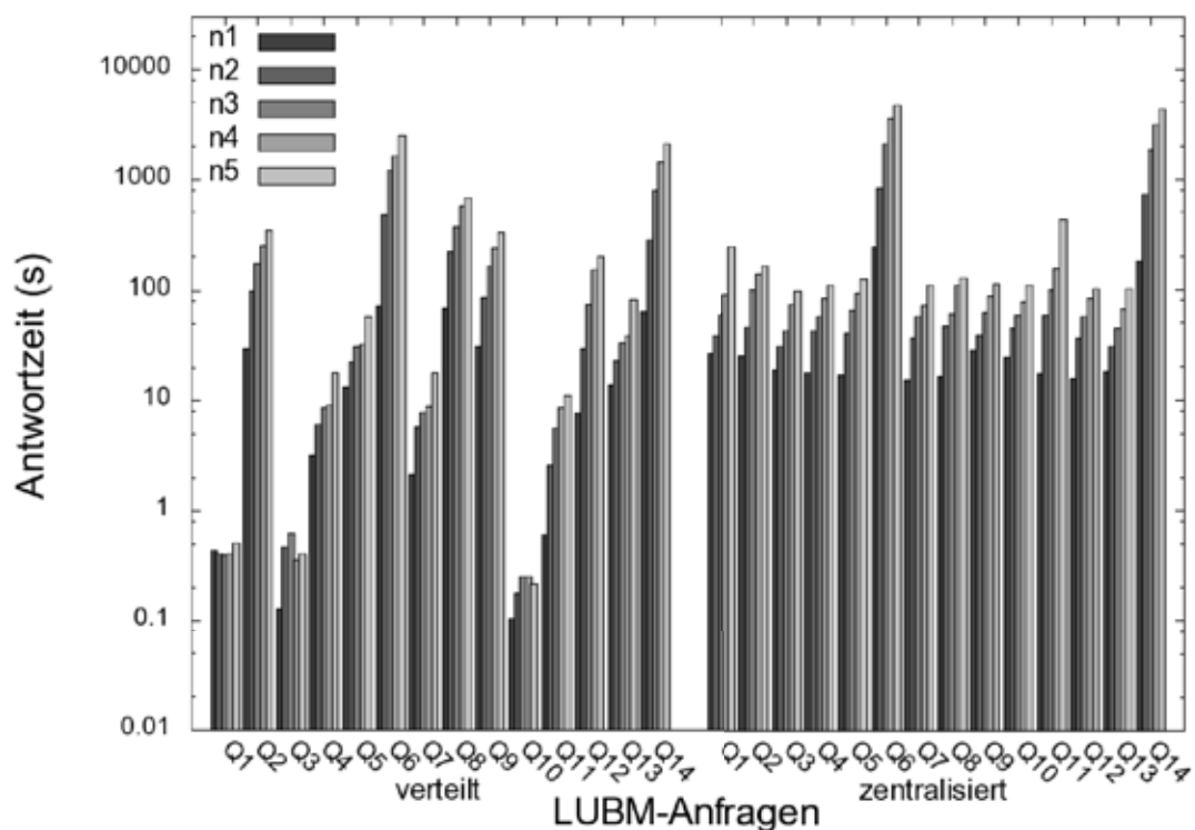
Abbildung A.1.: Gegenüberstellung der Antwortzeiten für alle LUBM-Test-Anfragen bei zwei Teil-Wissensbasen.
