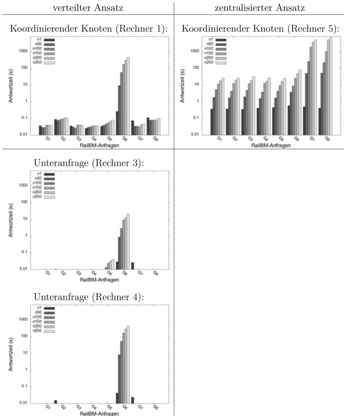
Abbildung 5.20.: Gegenüberstellung der Antwortzeiten für die RAILBM-Anfragen im verteilten (links) und zentralisierten Fall (rechts) mit steigender Größe der Wissensbasen. Für den verteilten Fall sind außerdem die Antwortzeiten für die beteiligten Knoten auf den Rechnern 3 und 4 dargestellt.
