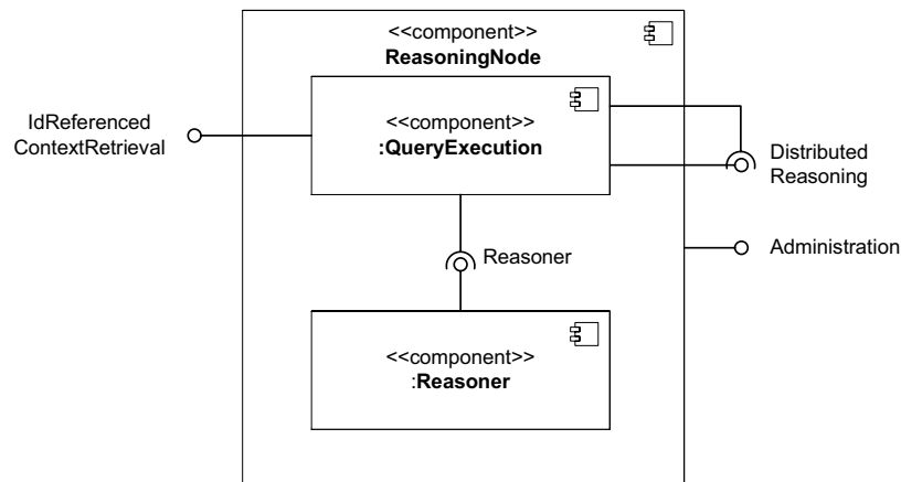
Abbildung 5.7.: Architektur der ReasoningNode-Komponente.
