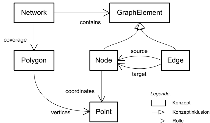
Abbildung 6.9.: Konzepte und Rollen zur beschreibungslogischen Repräsentation räumlicher Netzwerke.
