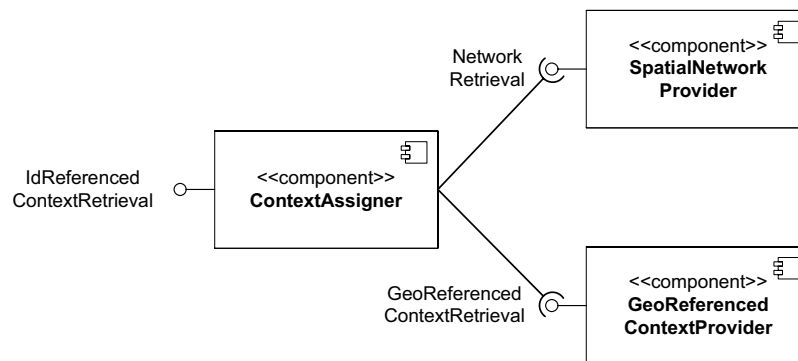
Abbildung 6.10.: Komponenten zur netzbasierten Integration ortsbezogener Kontextinformationen.
