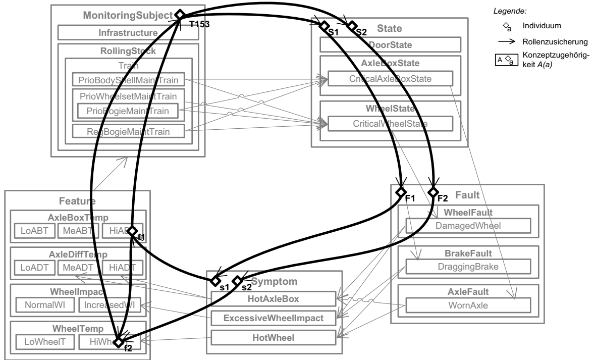
Abbildung 4.6.: Explizite Zusicherungen in der Wissensbasis.
