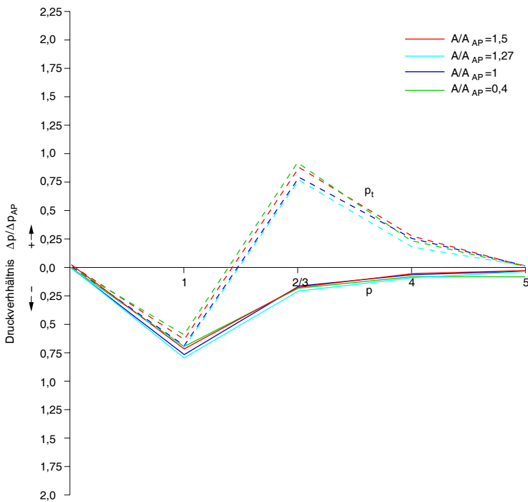
Abbildung 4.32: Verlauf des Druckverhältnisses \Delta p_{(t)}/\Delta p_{1,AP} an den Messstellen 0-5 für eine Drehzahl von 18000 \text{ min}^{-1} und einen Volumenstromverhältnis von \dot{V}/\dot{V}_{AP} = 1,0
