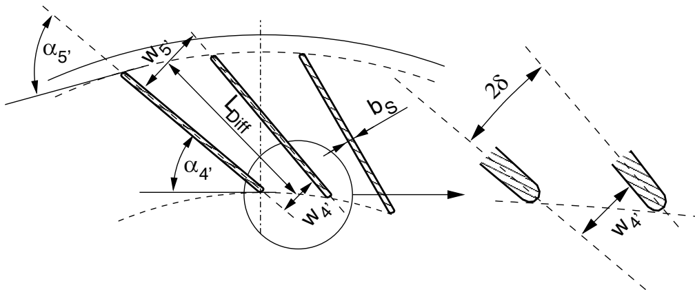
Abbildung 3.15: Verhältnisse der Teilbeschaufelung des Diffusors
