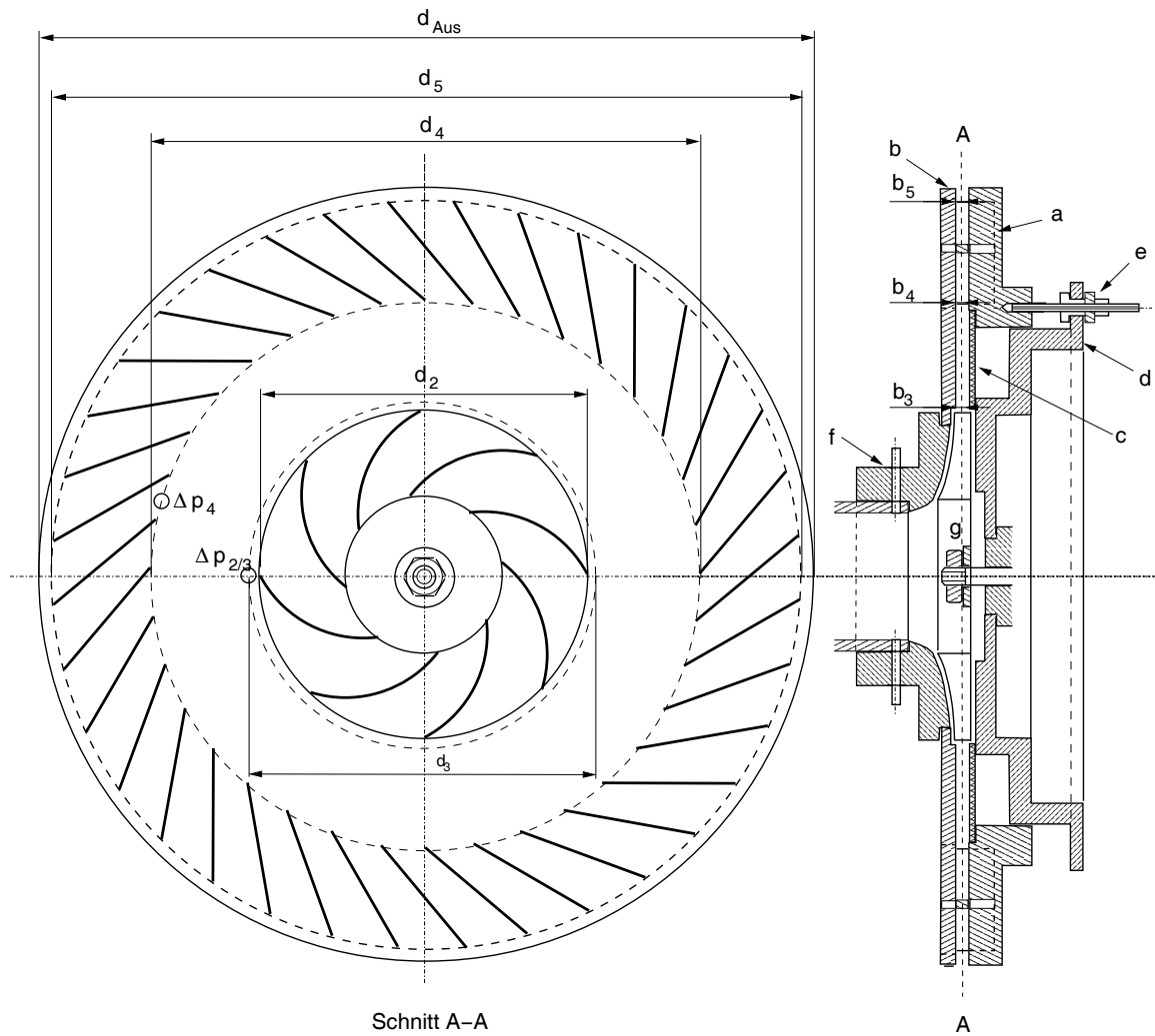
Abbildung 3.14: Radialgebläse mit teilbeschaufeltem, verstellbarem 48^\circ -Diffusor
