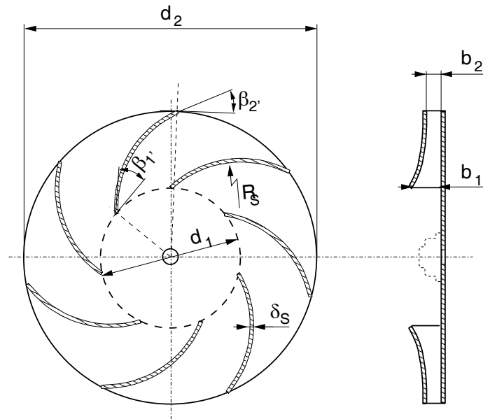
Abbildung 3.5: Laufrad des verwendeten Gebläses
