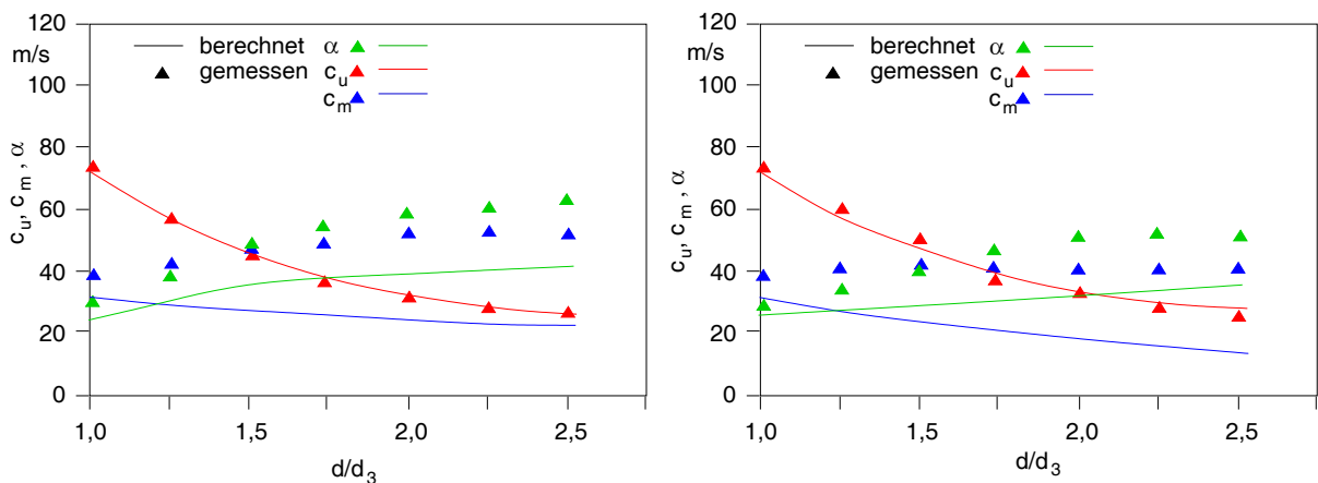
Abbildung 4.5: Verlauf der Geschwindigkeitskomponenten c_m und c_u und des Strömungswinkels \alpha für den parallelen Diffusor (links) und den um 3 mm aufgeweiteten Diffusor (rechts) bei n = 24000 \text{ min}^{-1} und \dot{V}/\dot{V}_{AP} = 1,6
