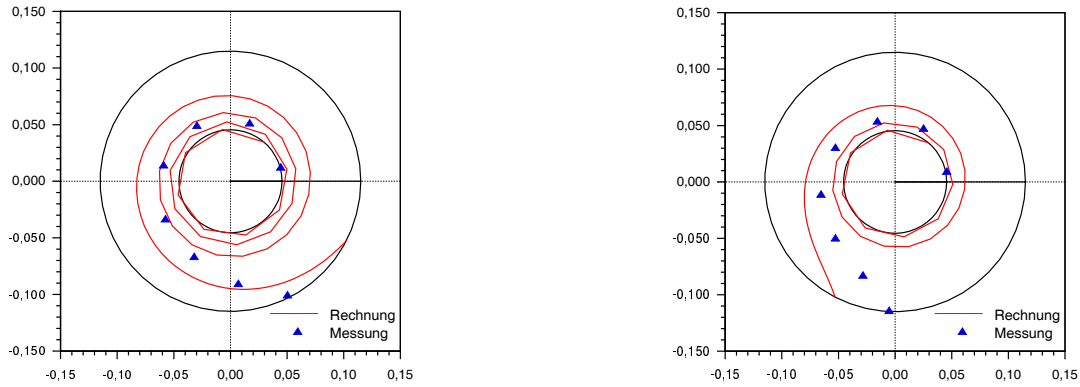
Abbildung 4.7: Vergleich einer berechneten Stromlinie mit den Messwerten für n = 24000 \text{ min}^{-1} , \dot{V}/\dot{V}_{AP} = 0,2 mit konvergentem \Delta b_4 = -4 \text{ mm} (rechts) und mit parallelem Diffusor (links)
