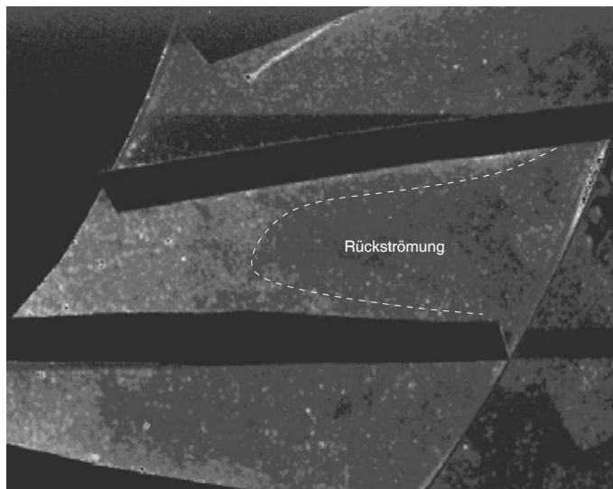
Abbildung 4.12: Partikelbild mit ausgeprägter Rückströmung in den Kanälen
