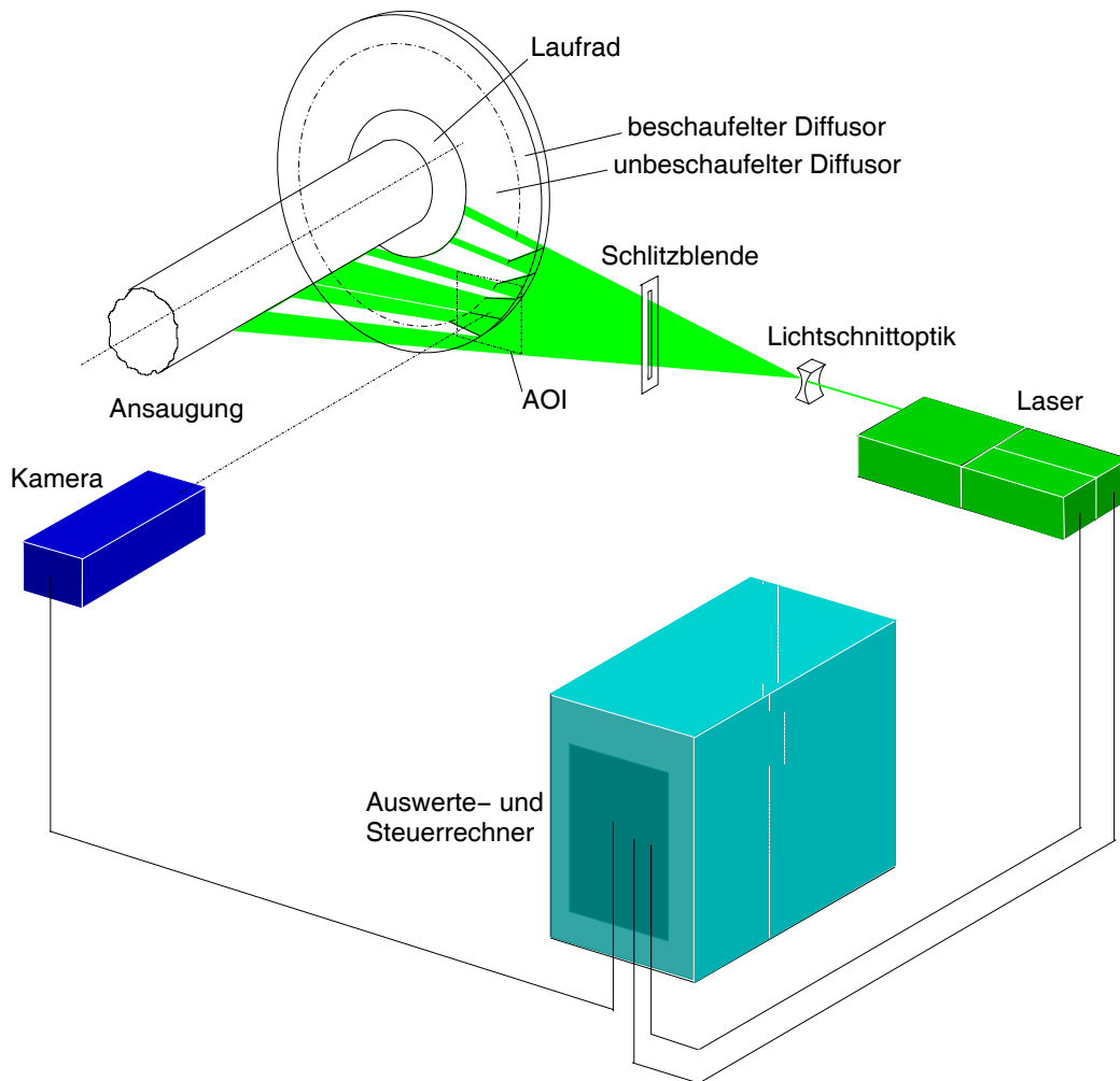
Abbildung 3.18: PIV Messaufbau bei beschaufeltem Diffusor
