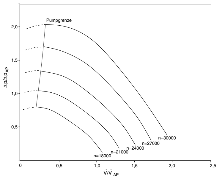
Abbildung 4.21: p-\dot{V} - Diagramm des Gebläses mit -4,5 mm verengtem Diffusor ( A_4/A_{4AP} \approx 0,18 )
