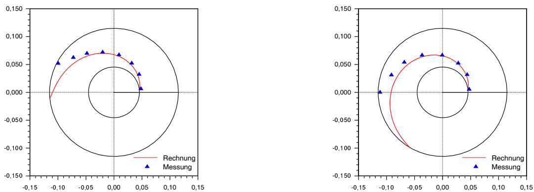
Abbildung 4.9: Vergleich einer berechneten Stromlinie mit den Messwerten für n = 24000 \text{ min}^{-1} , \dot{V}/\dot{V}_{AP} = 1,6 mit konvergentem \Delta b_4 = +3 \text{ mm} (rechts) und parallelem Diffusor (links).
