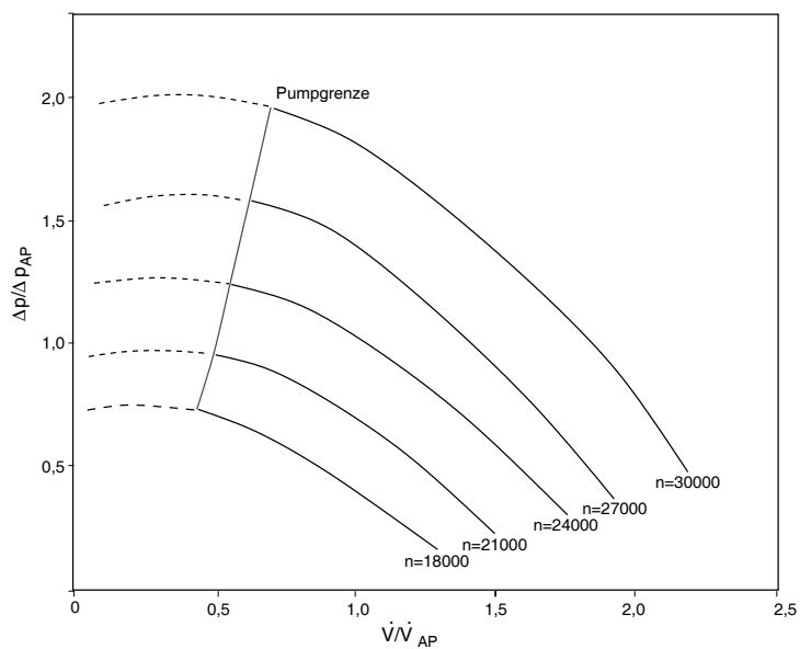
Abbildung 4.20: p-\dot{V} - Diagramm des Gebläses mit -3 mm verengtem Diffusor ( A_4/A_{4AP} \approx 0,27 )
