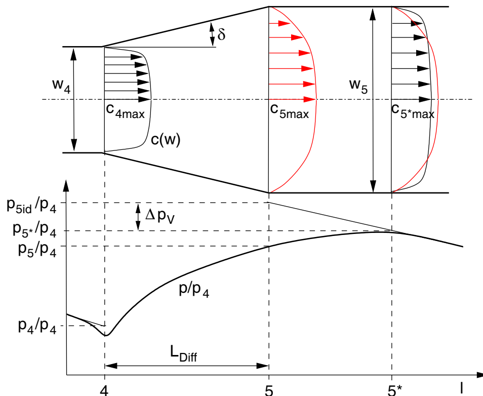
Abbildung 2.25: Verzerrung des Geschwindigkeitsprofils am Austritt des Diffusors und Ausgleich im Nachlauf, sowie Verlauf des auf den Eintrittszustand bezogenen Druckes über der Diffusorlänge mit Vor- und Nachlauf
