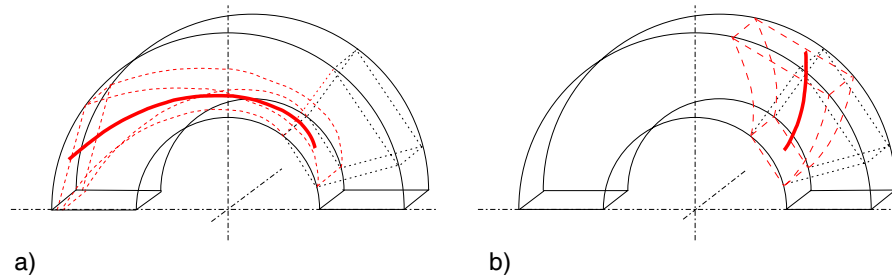
Abbildung 2.15: Stromlinie und „Diffusorkanal“ (gestrichelt) für niedrige (a) und hohe Volumenströme (b) sowie punktiert für einen radialesegmentierten Kanal eines „ebenen“ Diffusors
