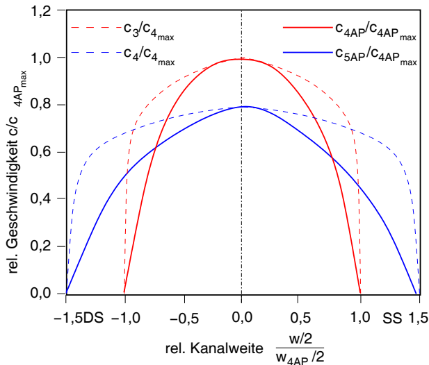
Abbildung 4.53: Verteilung der Geschwindigkeiten über den Querschnitt des parallelwandigen Diffusors aus den volumenstromgemittelten Geschwindigkeitsverteilungen der Vektorbilder 4.43 und 4.44 (ausgezogen) sowie die Verteilung für eine Kanalströmung nach dem 1/7-Potenzgesetz (gestrichelt)
