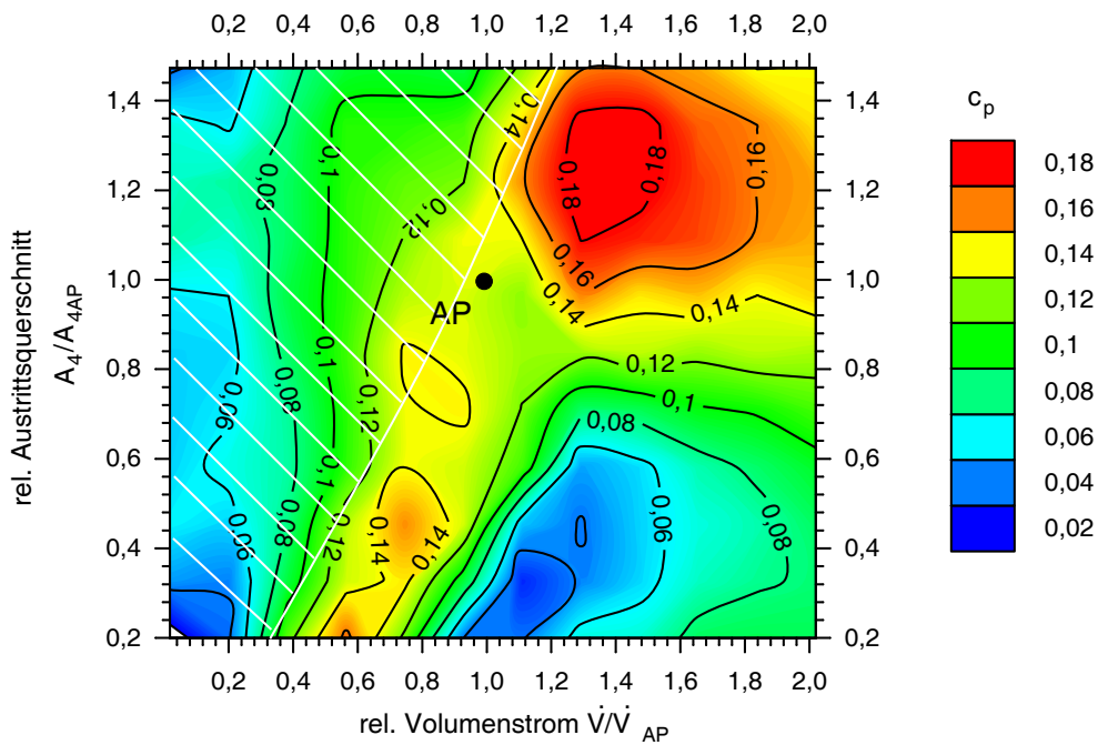
Abbildung 4.40: Verlauf des Diffusor-Druckbeiwertes des unbeschaufelten Diffusorteils c_{p_{3 \rightarrow 4}} in Abhängigkeit des Volumenstrom- und Querschnittsverhältnisses
