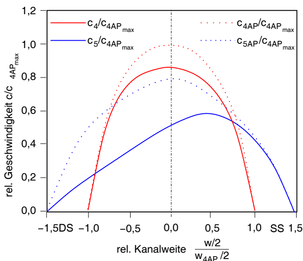
Abbildung 4.55: Verteilung der Geschwindigkeiten über den Querschnitt aus den volumenstromgemittelten Geschwindigkeitsverteilungen der Vektorbilder 4.48 bis 4.50 ( A_4/A_{4AP} \approx 1,95 ) sowie ausgezogen das gemessene Profil des parallelen Diffusors der Abb. 4.53 punktiert)
