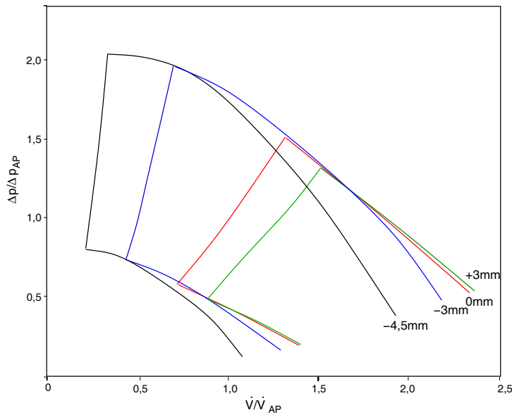
Abbildung 4.22: Vergleich der Arbeitsbereiche des Gebläses für Breitenveränderungen von -4,5 mm bis +3 mm ( A_4/A_{4AP} \approx 0,18 - 1,55 ).
