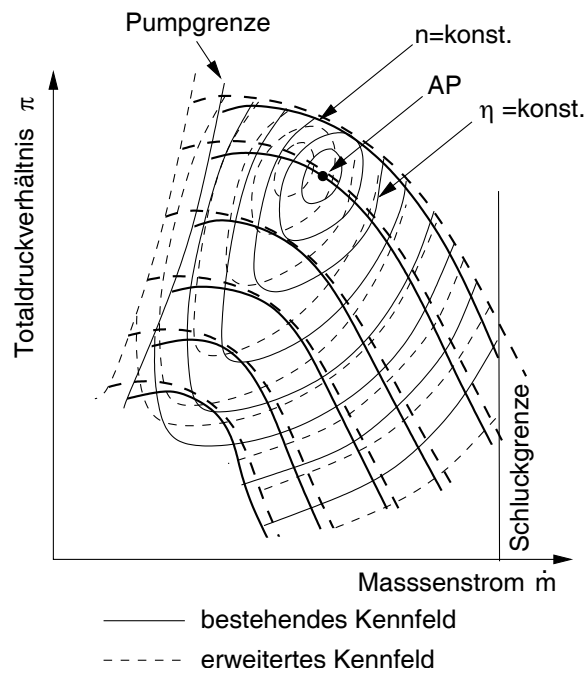
Abbildung 1.2: Kennfeld eines Radialgebläses mit Optimierungsziel
