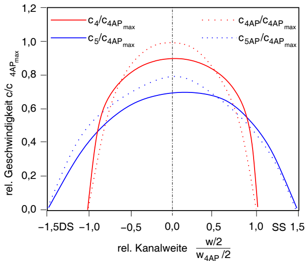
Abbildung 4.54: Verteilung der Geschwindigkeiten über den Querschnitt aus den volumenstromgemittelten Geschwindigkeitsverteilungen der Vektorbilder 4.45 bis 4.47 ( A_4/A_{4AP} \approx 1,55 ) sowie ausgezogen das gemessene Profil des parallelen Diffusors der Abb. 4.53 punktiert)
