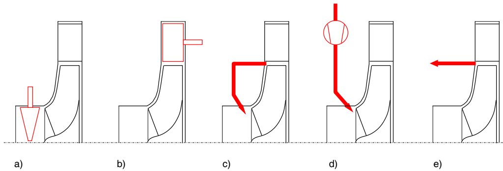
Abbildung 2.32: Strategien zur Vermeidung eines Strömungsabrisses durch a) Drallaufprägung durch Vorleitbeschaukelung, b) Leitschaukelverstellung, c) Rückführung, d) konstante oder gepulste Einblasung von Fremdluft und e) Abblaseeinrichtung
