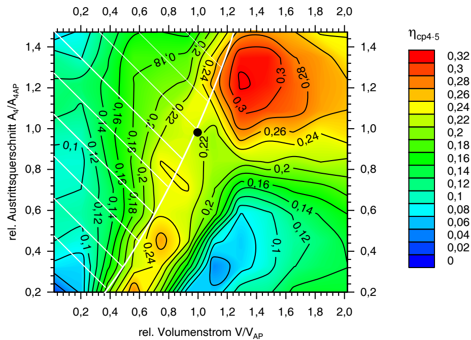
Abbildung 4.42: Diffusor-Gütegrad des beschaukelten Diffusorteils \eta_{Diff_{4 \rightarrow 5}} in Abhängigkeit des Volumenstrom- und Querschnittsverhältnisses
