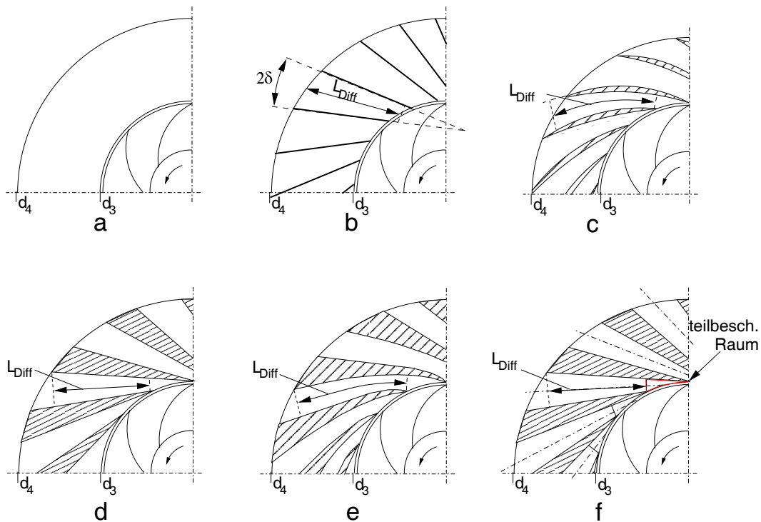
Abbildung 2.9: Diffusorbauarten: a) unbeschaufelt, b) gerade Schaufel, c) Profilschaukel, d) Keilschaukel, e) Vane-Island-Schaukel, f) Rohrkanal-Diffusor nach [27] ( L_{Diff} : wirksame Diffusorlänge; 2\delta : Diffusoröffnungswinkel )
