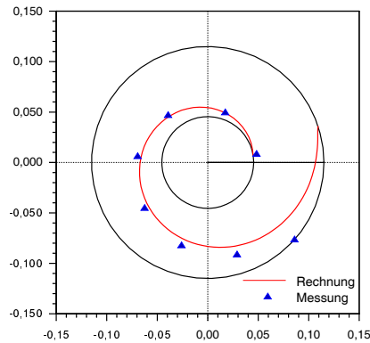
Abbildung 4.8: Vergleich einer berechneten Stromlinie mit den Messwerten für n = 24000 \text{ min}^{-1} , \dot{V} = \dot{V}_{AP} bei parallelem Diffusor
