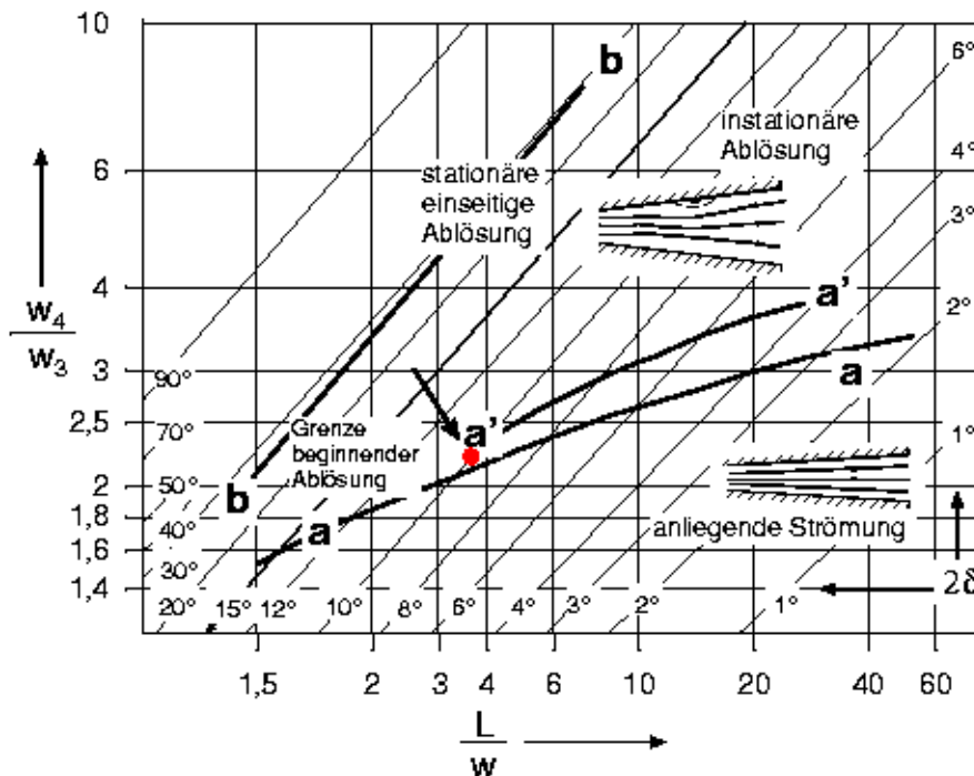
Abbildung 3.17: Einordnung des beschaufelten Diffusors in das Diffusordigramm nach COCKRELL bzw. FOX und KLINE
