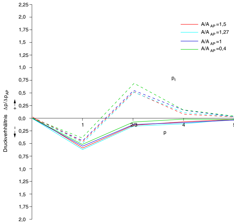
Abbildung 4.35: Verlauf des Druckverhältnisses \Delta p/\Delta p_{1_{AP}} sowie des Totaldruckverhältnisses \Delta p_t/\Delta p_{t1_{AP}} an den Messstellen 0-5 für eine Drehzahl von 24000 \text{ min}^{-1} und ein Volumenstromverhältnis von \dot{V}/\dot{V}_{AP} = 1,8
