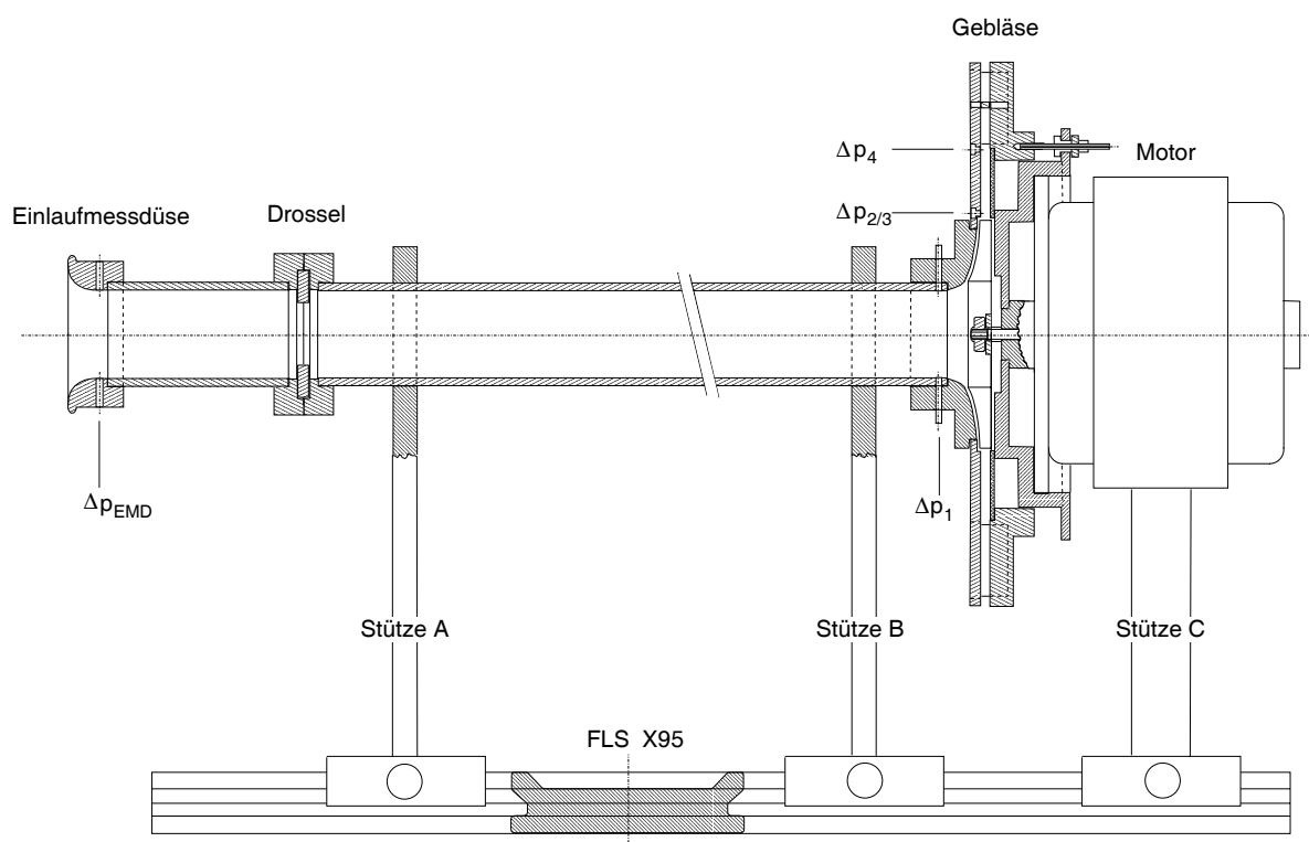
Abbildung 3.1: Aufbau des Gebläseversuchsstandes mit beschaufeltem Gebläse und Anordnung der Druckmessstellen
