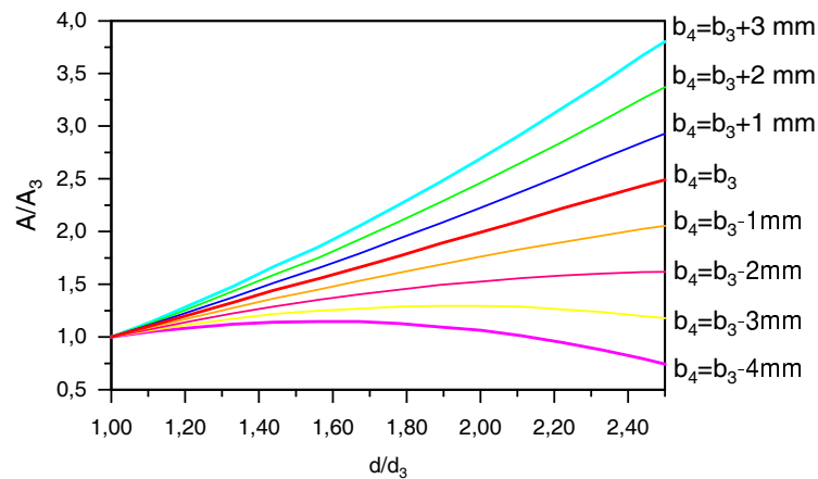
Abbildung 3.9: Änderung des Strömungsquerschnittes zwischen Diffusorein- und Diffusoraustritt für Breitenänderungen von -4 bis +3mm
