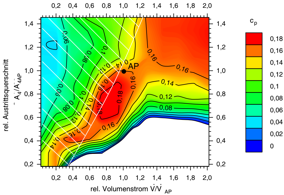
Abbildung 4.40: Verlauf des Diffusor-Druckbeiwertes des unbeschaufelten Diffusorteils c_{p_{3 \rightarrow 4}} in Abhängigkeit des Volumenstrom- und Querschnittsverhältnisses
