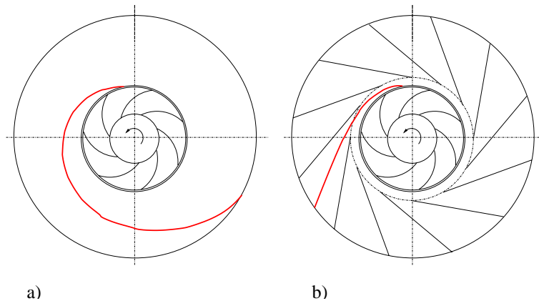
Abbildung 2.10: Stromlinie im unbeschaukelten (a) bzw. beschaukelten Diffusor (b)
