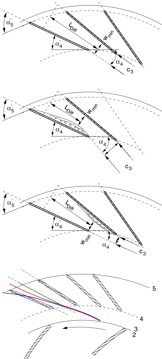
Abbildung 2.20: Anströmung des Diffusors im Auslegungsfall (oben) bei Volumenströmen oberhalb des Auslegungsfalles (Bruststoß, mittig) und unterhalb des Auslegungsfalles (Nackenstoß, unten)
