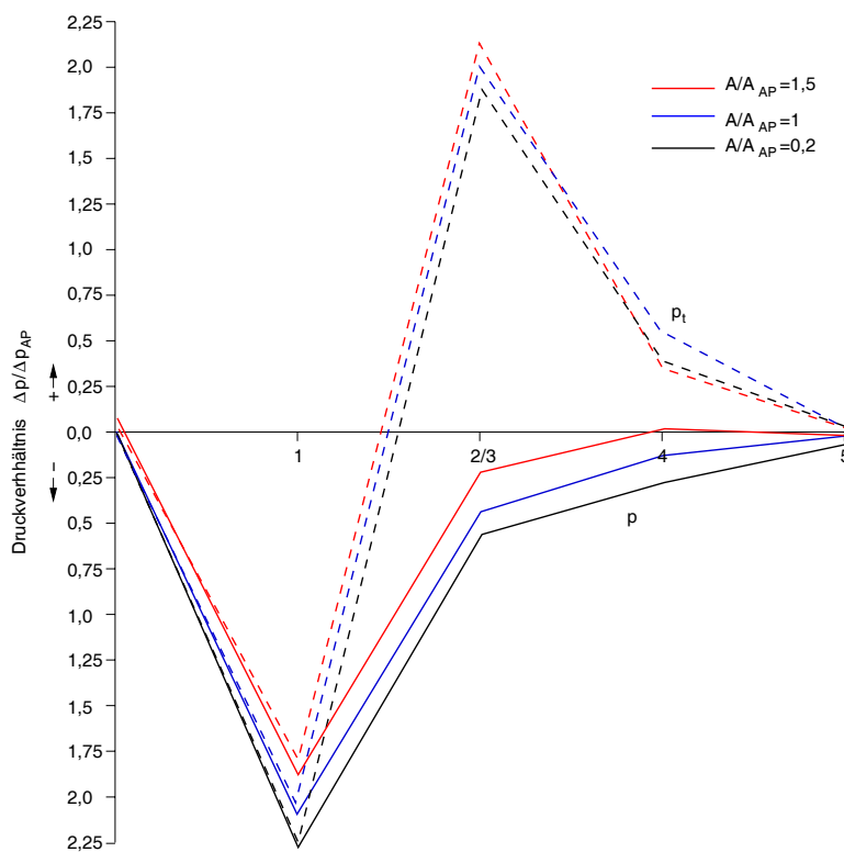
Abbildung 4.36: Verlauf des Druckverhältnisses \Delta p/\Delta p_{1_{AP}} sowie des Totaldruckverhältnisses \Delta p_t/\Delta p_{t1_{AP}} an den Messstellen 0-5 für eine Drehzahl von 30000 \text{ min}^{-1} und ein Volumenstromverhältnis von \dot{V}/\dot{V}_{AP} = 0,2
