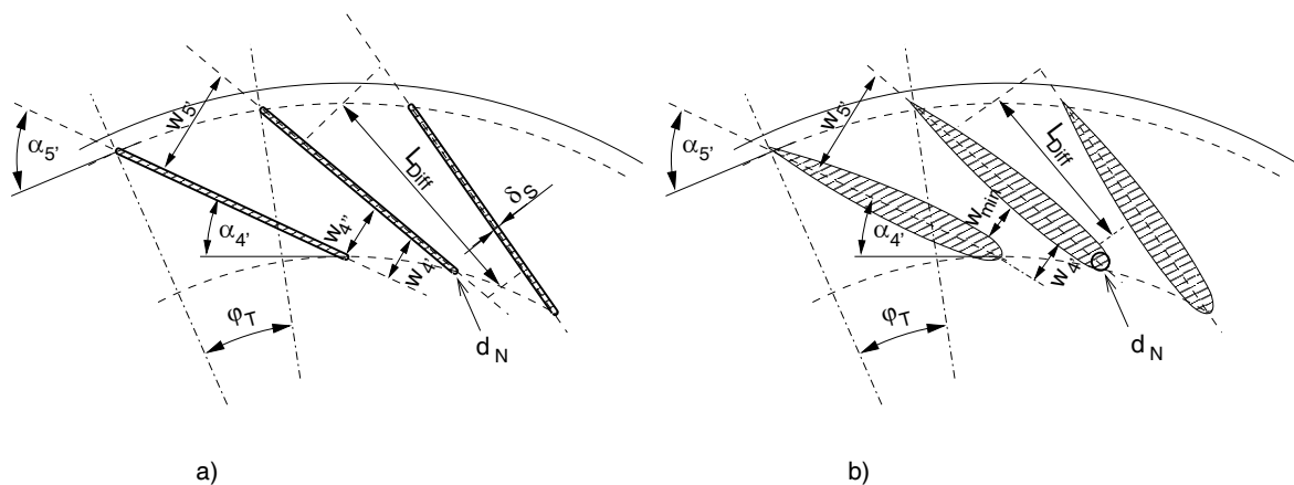
Abbildung 2.19: a) Plattendiffusor mit kleinem Nasendurchmesser d_N und dünnen Schaukeln b) Diffusor mit großem Nasendurchmesser d_N und profilierten Schaukeln
