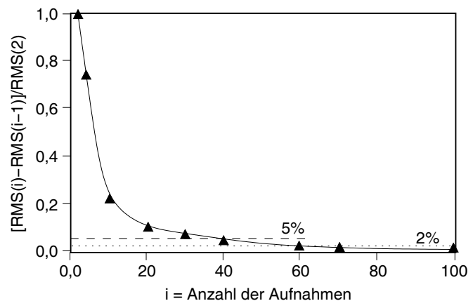
Abbildung 3.13: Verlauf der bezogenen Änderung des RMS-Wertes über der Anzahl der Aufnahmen i
