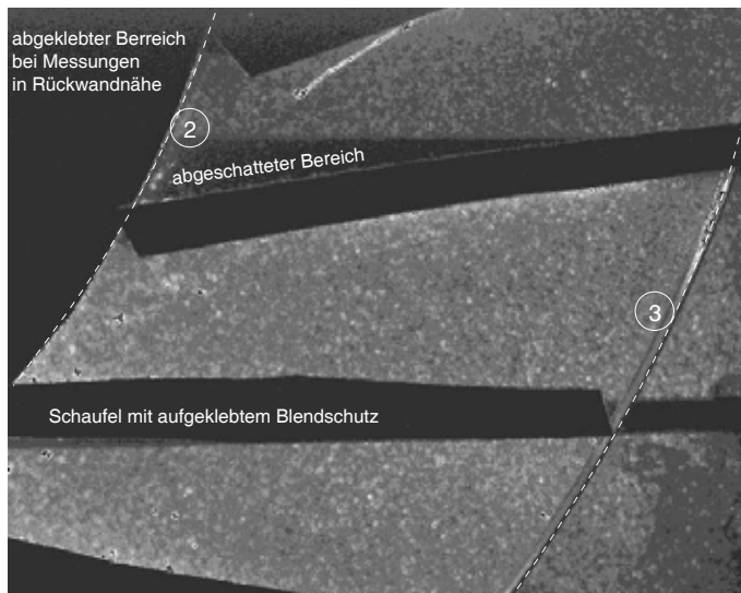
Abbildung 4.11: Partikelbild einer vollausgebildeten Diffusorströmung
