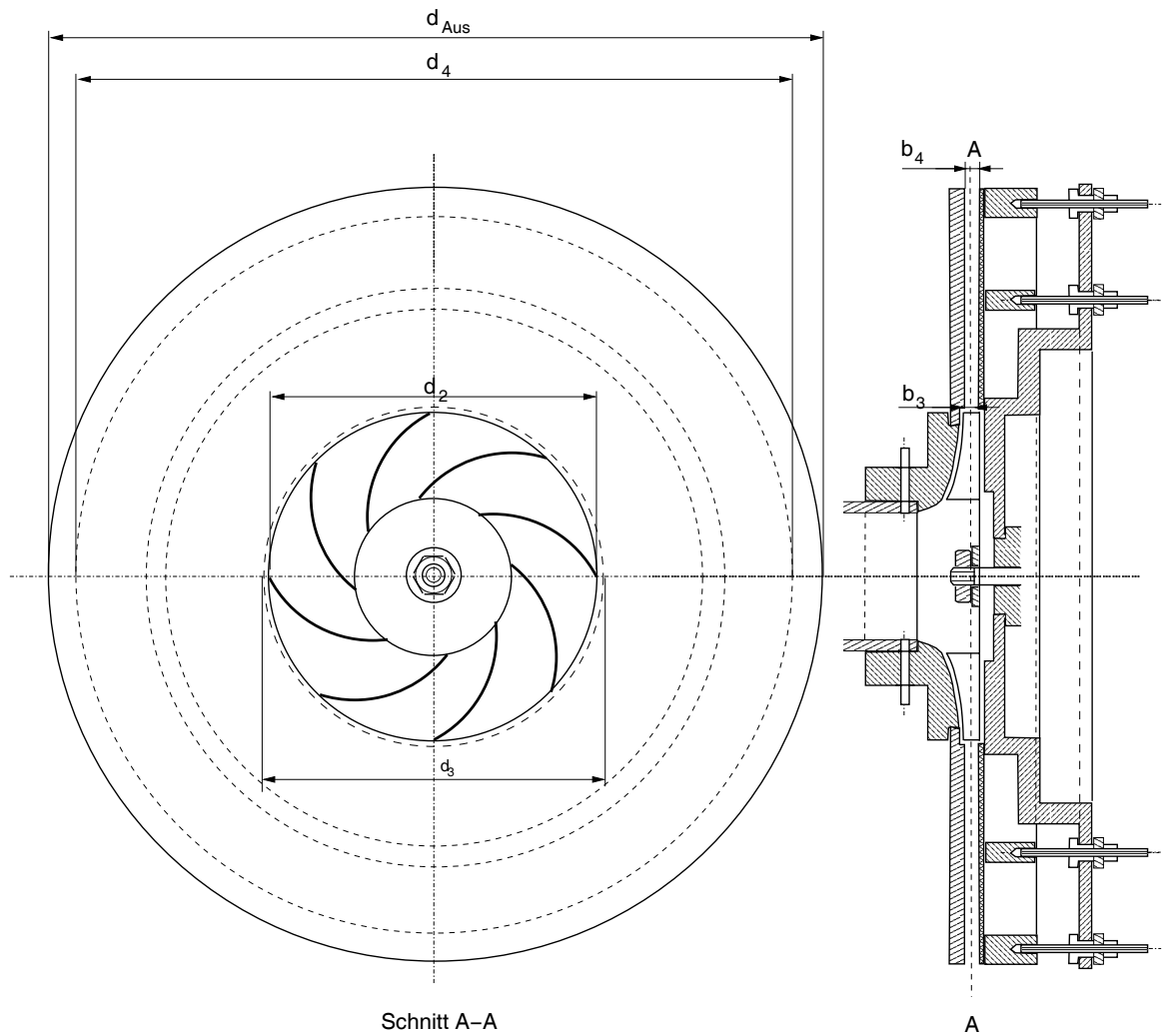
Abbildung 3.7: Der unbeschaufelte Diffusor
