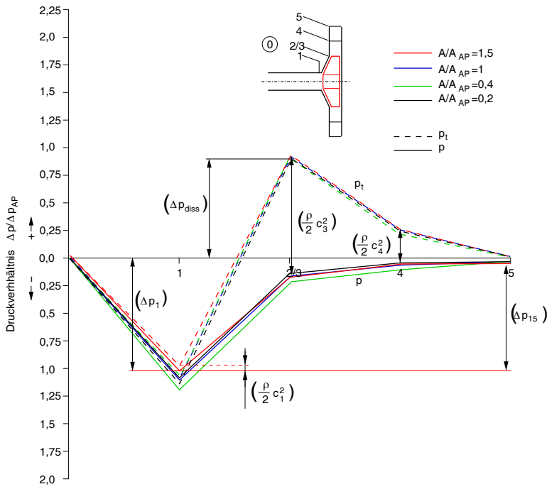
Abbildung 4.31: Verlauf des Druckverhältnisses \Delta p_{(t)}/\Delta p_{1,AP} an den Messstellen 0-5 für eine Drehzahl von 18000 \text{ min}^{-1} und einen Volumenstromverhältnis von \dot{V}/\dot{V}_{AP} = 0,2
