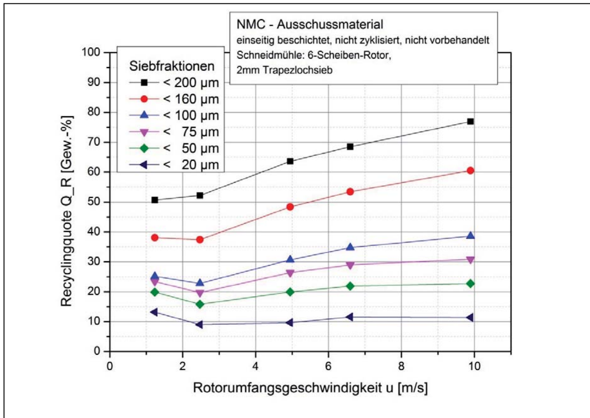
Abbildung B-23: Anteil der Feinfraktionen nach Beanspruchung in Schneidmühlen bei variierter Rotordrehzahl für die Klassierung (Siebung) bei verschiedenen Trennkorngrößen (6-Scheiben-Rotor, 2mm Trapezlochsieb)
