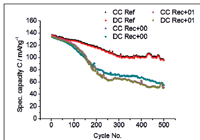
Abbildung D-2: Zyklisierkurve von NMC bei 40°C
