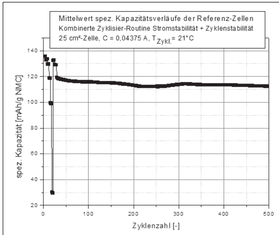
Abbildung C-6: Elektrochemischer Zyklientest einer Referenzzelle aus Neumaterialien – Stromstabilitätstest (Zyklen 1-30) und Zyklenstabilität bei 3C (Zyklen 30-500)
