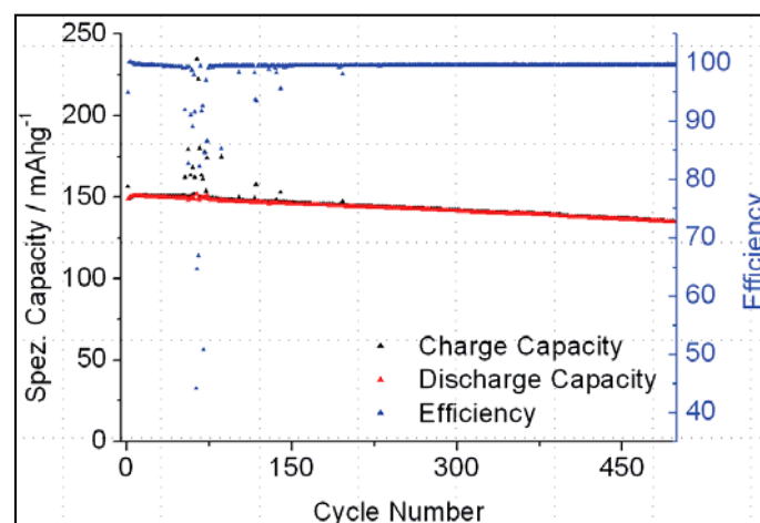
Abbildung D-1: Zyklisierkurve von LiFePO 4 bei 40°C
