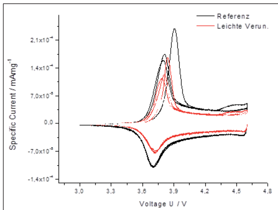
Abbildung C-12: CV Test
