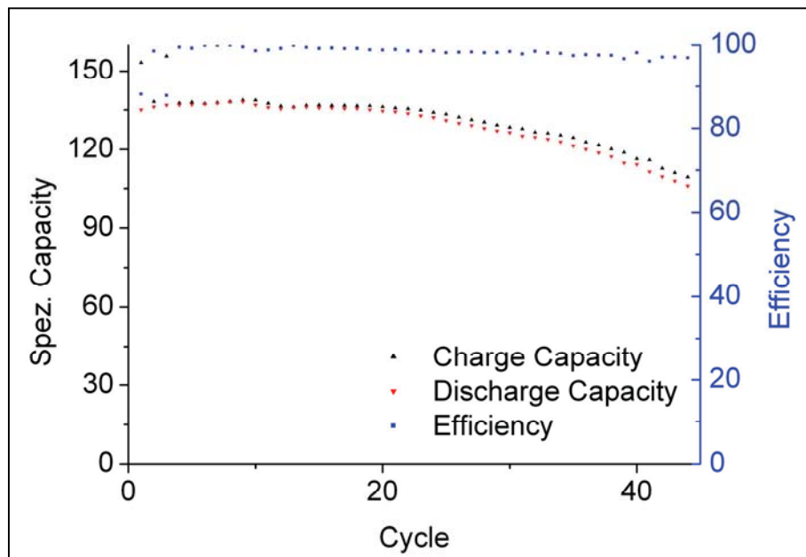
Abbildungung C-4: Zyklierungskurve von LiFePO 4 bei Raumtemperatur
