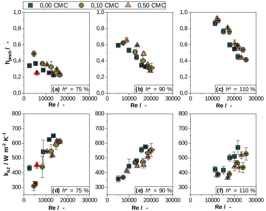
Abbildung 38: Länge der Aufheizzone h_{\text{pinch}} und Wärmedurchgangskoeffizient in der Aufheizzone k_{Az} in Abhängigkeit der Reynolds-Zahl Re für scheinbare Füllstände von 75 %, 90 % und 110 %, Tensidanteile von 0,0 CMC, 0,1 CMC und 0,5 CMC und einem Betriebsdruck p = 700 mbar
