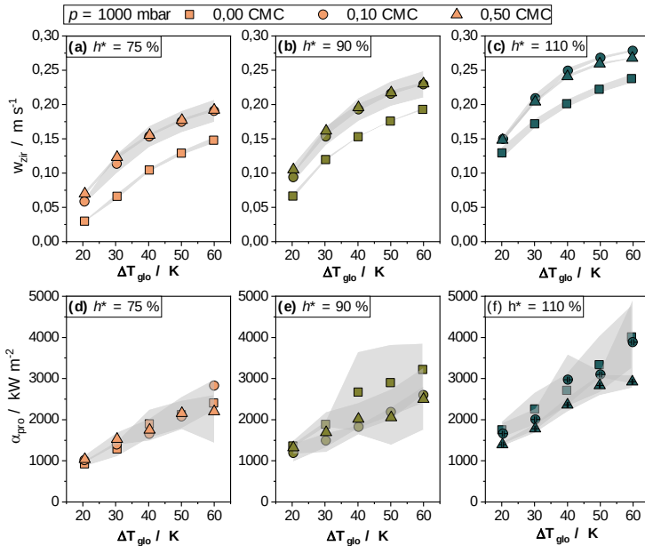
Abbildung 58: Beeinflussung des integralen Betriebsverhalten des Naturumlaufverdampfers durch die Zugabe von SAS für einen Betriebsdruck von 1.000 \text{ mbar} . Dargestellt sind die Umlaufgeschwindigkeit sowie der produktseitige Wärmeübergangskoeffizient in Abhängigkeit der treibenden Temperaturdifferenz für variierende scheinbare Füllstände und massebezogene Tensidanteile.
