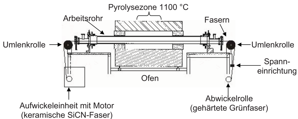
Abb.13: Schema des verwendeten Pyrolyseofen zur kontinuierlichen Herstellung keramischer SiCN-Fasern.
