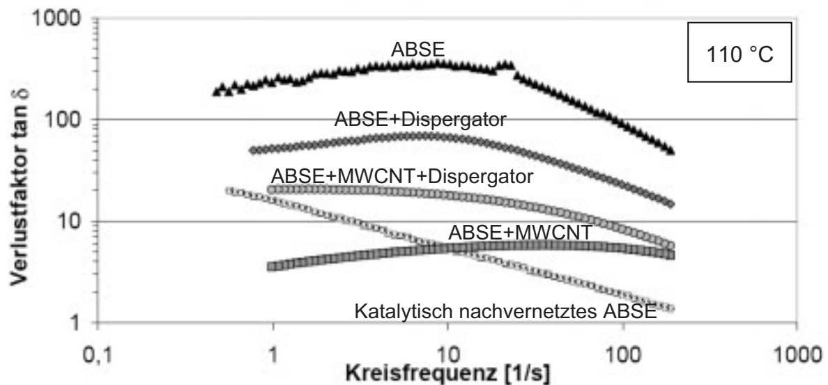
Abb. 27: Verlauf des Verlustfaktors \tan \delta bei 110\text{ °C} über der Kreisfrequenz, Untersuchung des Einflusses der Zugabe von 1 Gew.% MWCNT und/oder 1 Gew.% Dispergator in den ABSE-Ausgangsprecursor.
