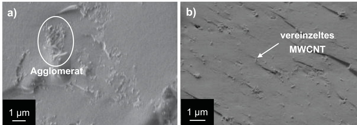
Abb. 22: a) Restagglomerate in der Größe von 2-5 \mu\text{m} ohne Verwendung eines Dispergators und b) homogen verteilte und vereinzelt MWCNT durch Verwendung eines Dispergators.
