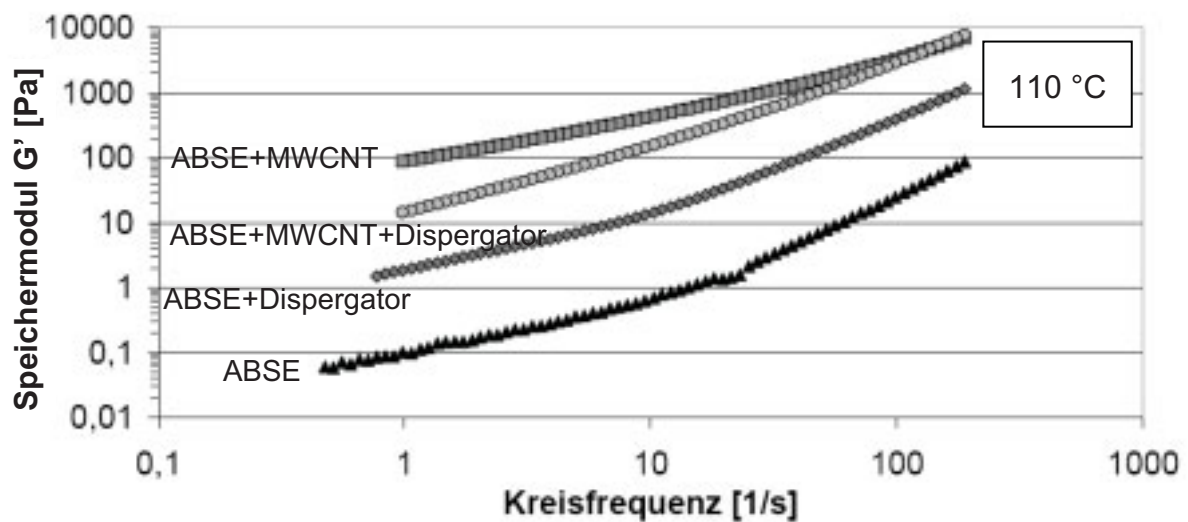
Abb. 28: Verlauf des Speichermoduls bei 110 °C über der Kreisfrequenz, Untersuchung des Einflusses durch Zugabe von 1 Gew.% MWCNT und/oder 1 Gew.% Dispergator in den Ausgangsprecursor.
