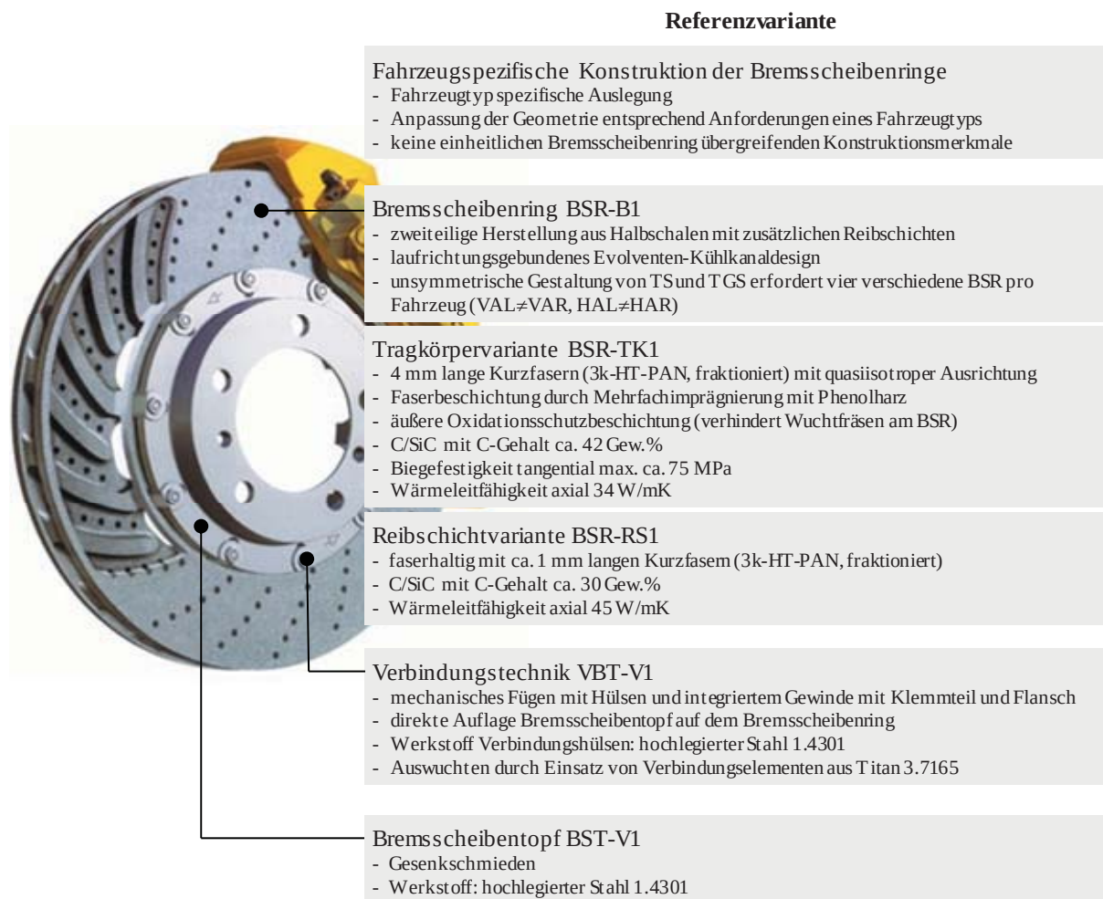
Abbildung 1-1: Referenzvariante in mehrteiliger Bauweise, bestehend aus dem Bremsscheibenring, dem Bremsscheibentopf und einzelnen Verbindungselementen.
