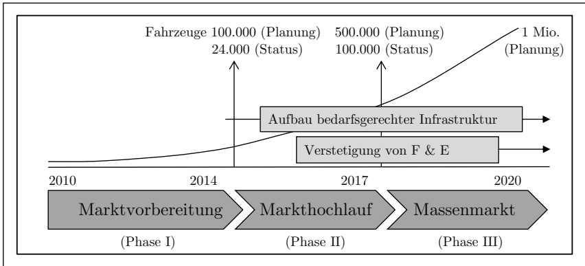
Abbildung 2-2: Entwicklungsphasen Elektromobilität
