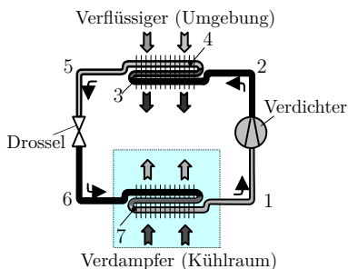
Abbildung 2.1: Prinzipskizze eines Kaldampfprozesses [WKW13].
