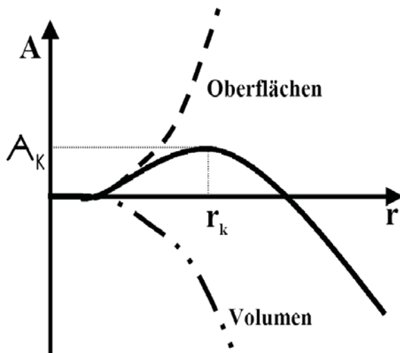
Abb. 2.3: Keimbildungsarbeit A in Abhängigkeit vom Radius r .
