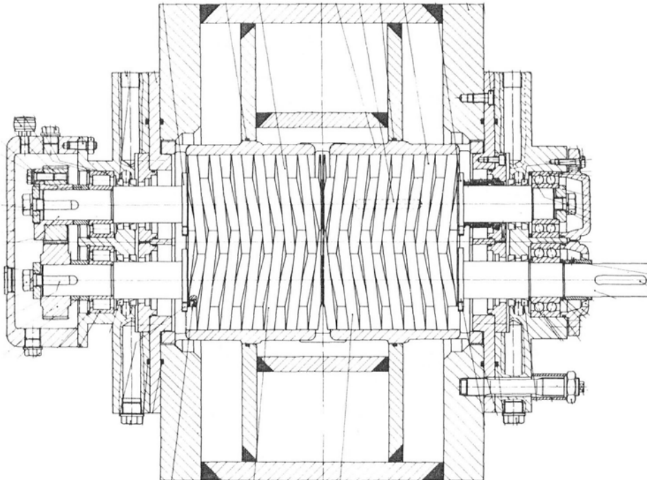
Bild 3.1: Zeichnung der von Vauth [4] eingesetzten Schraubenspindelpumpe
