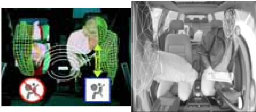
Abbildung 1.3: Im linken Bild wird die Unterscheidung zwischen Person und Kindersitz dargestellt (Personenklassifikation). Im rechten Bild wird eine Entfernungsmessung über die Position des Kopfes durchgeführt. Diese Ergebnisse wurde mit einem System der Firma Robert-Bosch erzeugt und in [A10] veröffentlicht. Bildquelle [A10]
