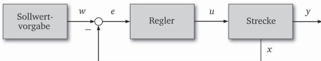
Bild 2.5: Struktur einer Regelung
